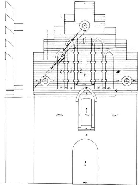
Fig. 6. Våbenhusets gavle 1:100. Formentlig tegnet o. 1906 af Carl Kiilsgaard. LAVib. - The gable of the porch.
