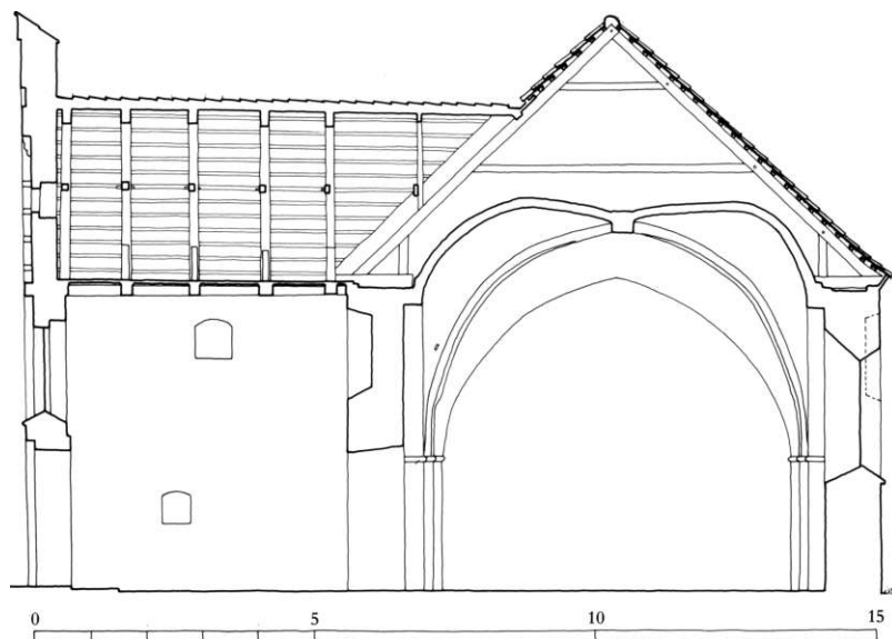
Fig. 8. Snit i våbenhus og skib 1:150. Målt af John Bennetzen 1992, tegnet af KdeFL 1997. - Section of the porch and the nave, looking east.
