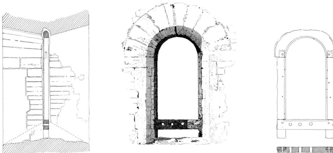
Fig. 9. Vindue og *ramme af egetræ 1:25. Korets nordside. Målt og tegnet af Valdemar Koch 1897. - Window and *frame of oak in the north side of the chancel.
