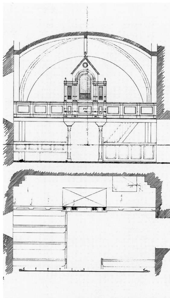
Fig. 35. Opstalt og plan af orgelpulpitur 1:125 (s. 4756). Carl Kiilsgaard 1907, LAVib. - Elevation and plan of organ loft.
