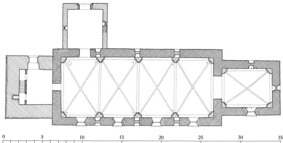
Fig. 7. Grundplan 1:300 tegnet af KdeFL 1997 efter Valdemar Koch 1897 og John Bennetzen 1992. - Ground-plan.
