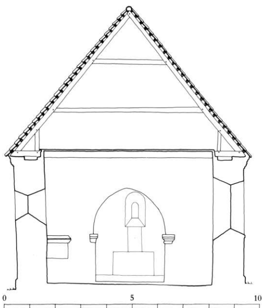
Fig. 9. Tværsnit i skibet set mod øst 1:150. Målt af Cathrine Gerner 1987, tegnet af KdeFL 1997. - Cross-section of the nave looking east.
