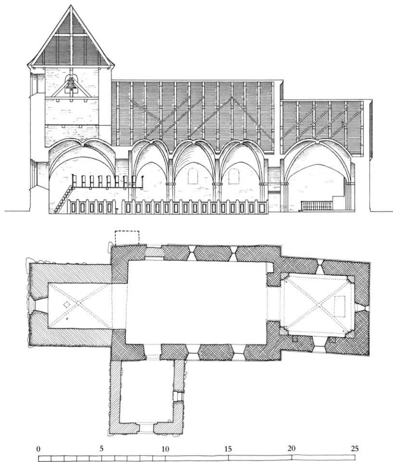
Fig. 3. Længdesnit og grundplan 1:300. Målt og tegnet henholdsvis ved Hector Estrup 1896 (før fjernelse af skibets hvælv), og af Cathrine Gerner 1987 og KdeFL 1997. - Longitudinal section and ground-plan.
