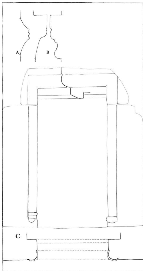
Fig. 4. Enkeltheder af granit, målt af Cathrine Gerner 1987, tegnet af KdeFL 1997. A. Overligger ved niche i triumfvæggen 1:15 (s. 4773). B. Korbuens vederlagsbånd 1:15 (s. 4773). C. Søndre portal 1:30 (s. 4772). - A. Moulded ashlar above niche in the east wall of nave. B. The imposts of the chancel arch. C. South portal.
