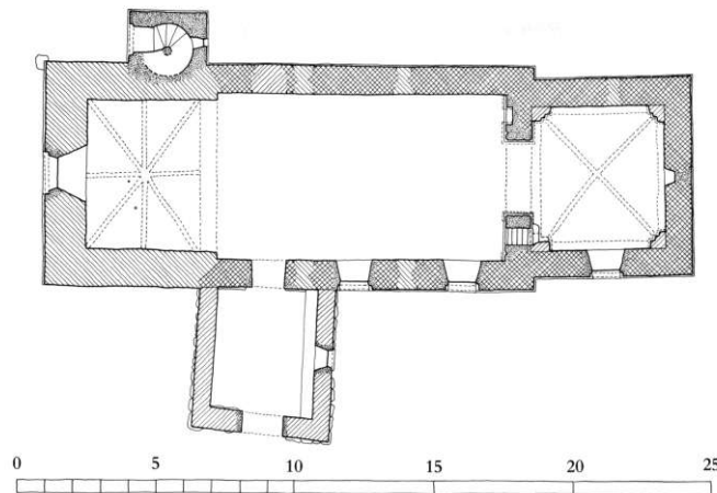
Fig. 4. Grundplan 1:300. Opmålt af Cathrine Gerner Hansen 1987, tegnet af KdeFL 1998. - Ground-plan.
