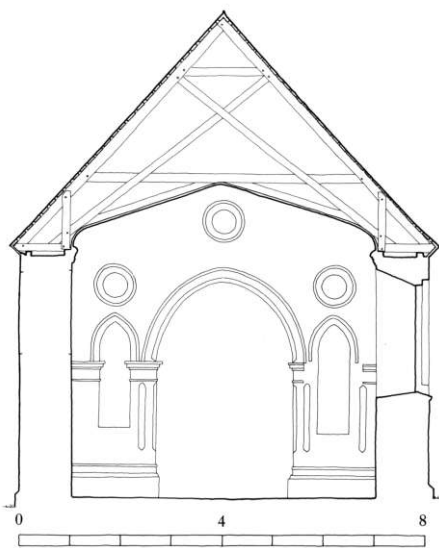
Fig. 5. Tværsnit i skibet set mod øst 1:150. Opmålt af Cathrine Gerner Hansen 1987, tegnet af KdeFL 1998. - Cross-section of the nave looking east.
