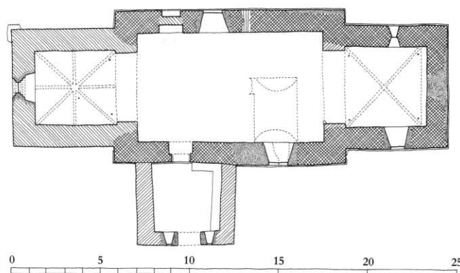
Fig. 4. Grundplan 1:300. Opmålt af Cathrine Gerner Hansen 1987, tegnet af KdeFL 1999. - Ground-plan.
