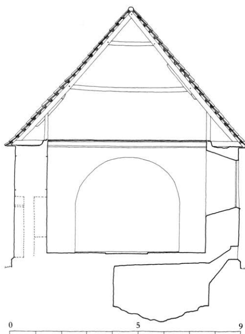
Fig. 5. Tværsnit i skibet set mod øst 1:150. Opmålt af Cathrine Gerner Hansen 1987, tegnet af KdeFL 1999. - Cross-section of the nave looking east
