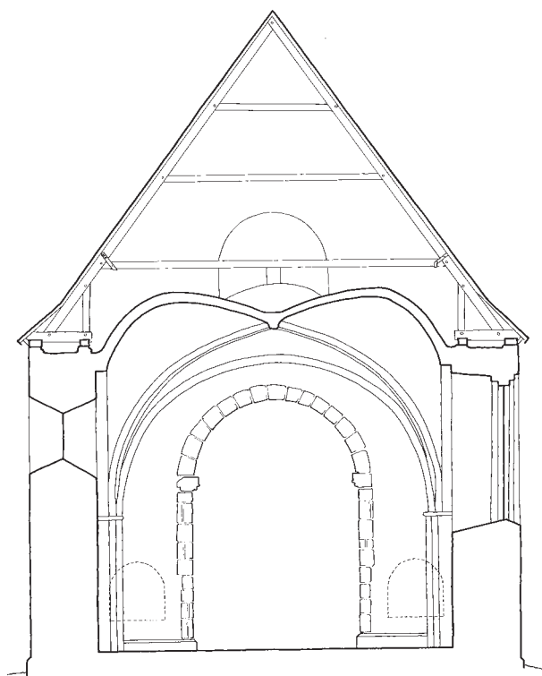
Fig. 4. Tværsnit 1:150 af skibet set mod øst. Tegnet 2002 af Marianne Nielsen efter opmåling af Peter Duun Andersen 2002, suppleret af Niels Jørgen Poulsen. – Cross-section of the nave looking east.
