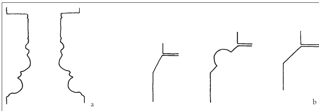
Fig. 53a-b. Romanske granitprofiler 1:10. a. Nordre og søndre korbuekragbånd, set mod øst (s. 5234). b. Sokkel under hhv. apsis, kor og skib (s. 5228). Målt af Peter Duun Andersen og Niels Jørgen Poulsen, tegnet af Marianne Nielsen 2002. — Romanesque granite profiles. a. Northern and southern chancel arch cordons looking east. b. Base under apse, chancel and nave respectively.
