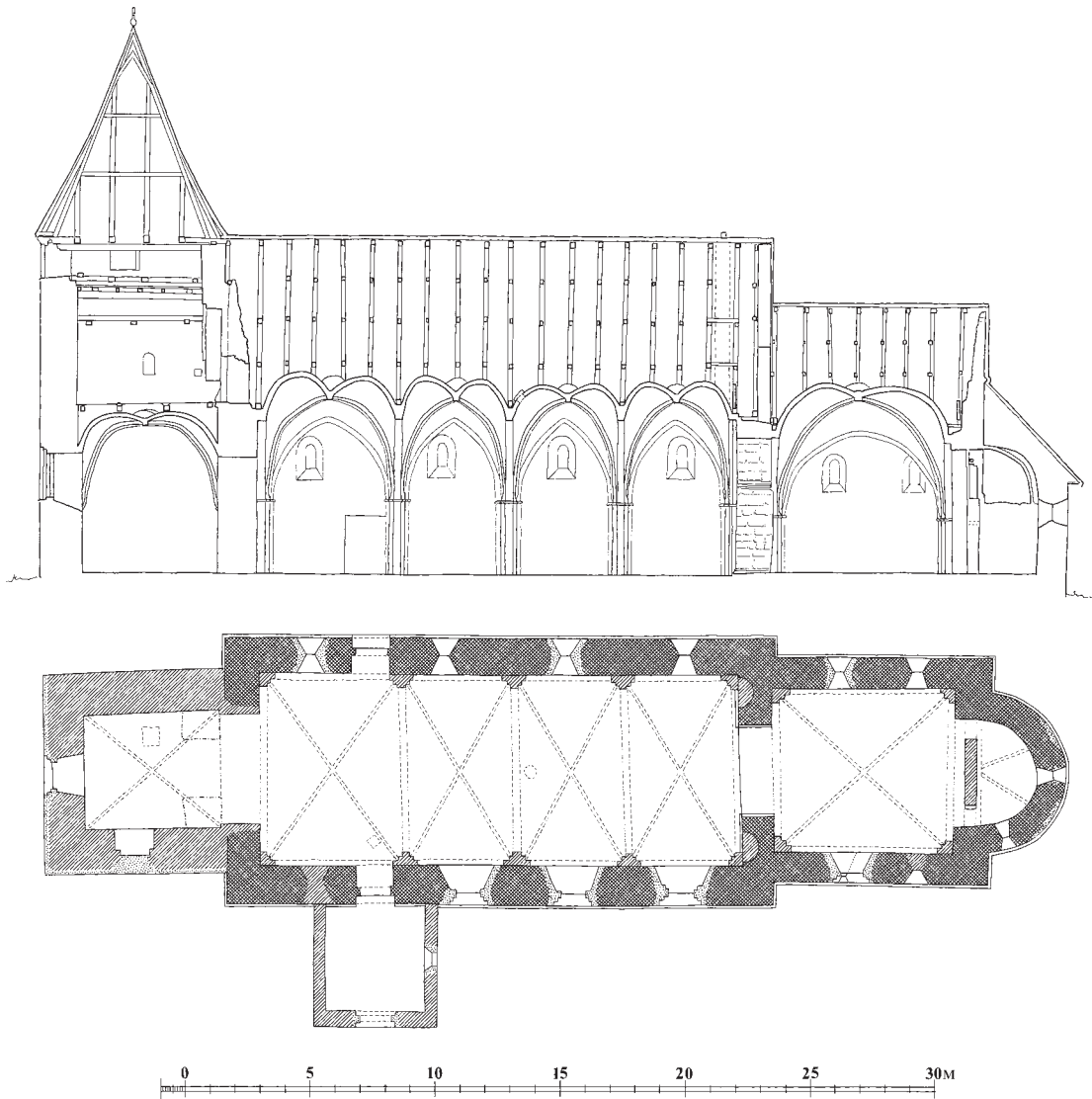
Fig. 5–6. Opmålinger 1:300. 5. Længdesnit af kirken. Tegnet 2002 af Marianne Nielsen efter opmåling af John Bennetzen 1990. 6. Plan. Tegnet 2002 af Marianne Nielsen efter opmåling af Mogens Clemmensen 1917 og Rolf Graae 1985, suppleret af Niels Jørgen Poulsen. – 5. Longitudinal section of the church . 6. Plan .
