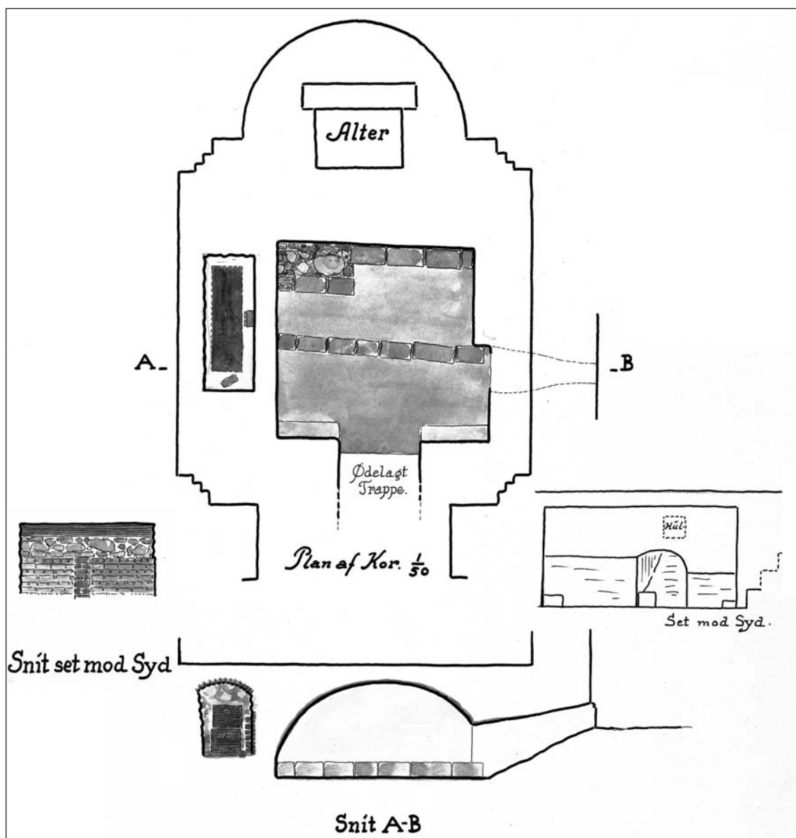
Fig. 48. Plan og snit af gravkrypt nr. 1 og 2 fra o. 1589 og derefter (s. 5261). 1:100. Farvelagt opmåling ved Peter Linde 1940. – Plan and section of Burial Crypts nos. 1 and 2 from c. 1589 and later.
