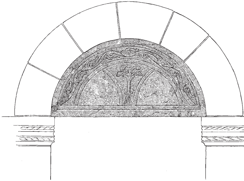
Fig. 52. Norddørens tympanon (s. 5233). 1:20. Jfr. fig. 12. Målt og tegnet af A. Claudi-Hansen 1912. — Tympanon of the north door. Cf. fig. 12.
