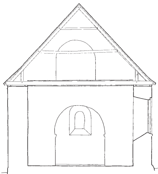
Fig. 4. Tværsnit 1:150 gennem skibet set mod øst. Målt af John Bennetzen 1991, tegnet af Marianne Nielsen 2002. – Cross-section through the nave looking east .
