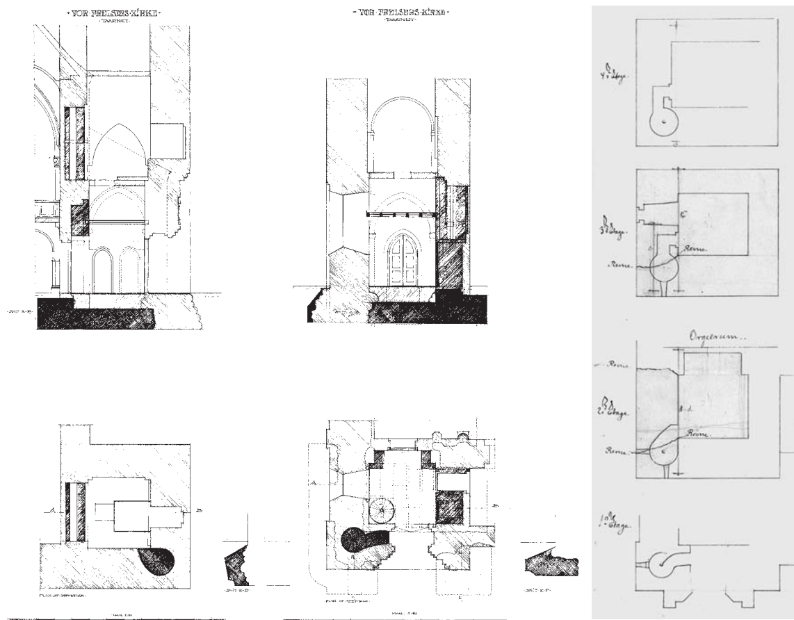
Fig. 68a-b. Opmålinger af tårnet. 1:300. a. Projekt til forstærkning af tårnets nedre stokværk (s. 5467). Tegnet af Viggo Norn 1924. b. Planer af tårnets stokværk med angivelse af revnedannelser (s. 5465). Skitse af Hector Estrup 1879. I Horsens Museum. — Surveys of the tower. 1:300. a. Project by Viggo Norn (1924) for reinforcing the lower storey. b. Plans of the storey with indications of crack formation. Sketch by Hector Estrup (1879).
