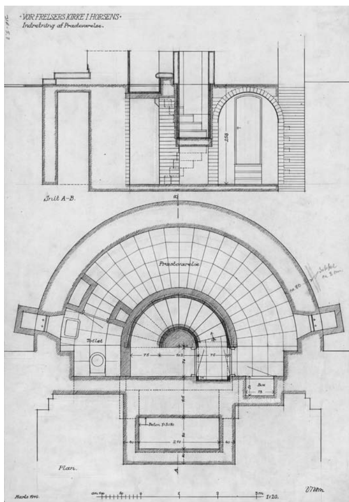
Fig. 86. Plan og snit af præsteværelse. 1:100. Tegnet af Viggo Norn 1949. I Horsens Museum. – Plan and cross-section of sacristy.
