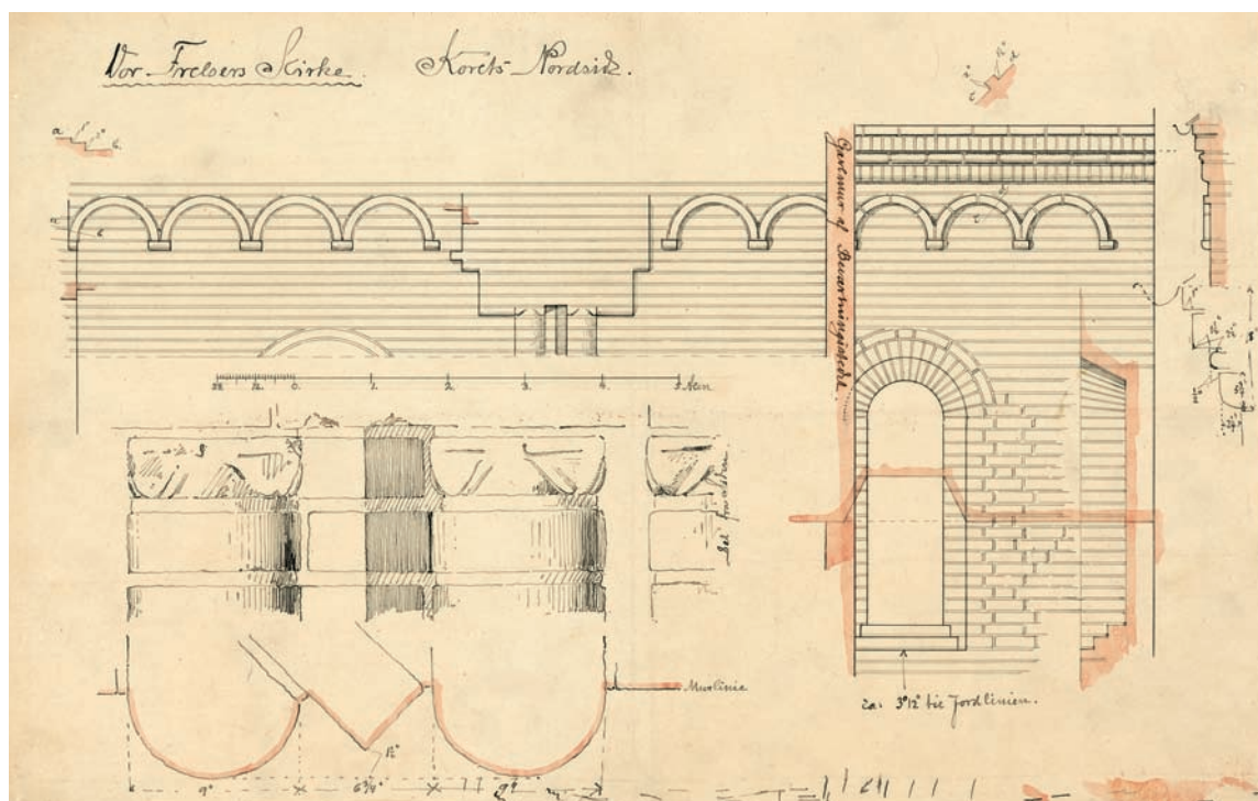
Fig. 33. Detaljer af korets nordside (s. 5404). Opmålingsblad ved Hector Estrup inden fjernelse af Tiltbygning 1879 (s. 5383). – Details of the north side of the chancel. Survey page before removal of Tannexe in 1879.
