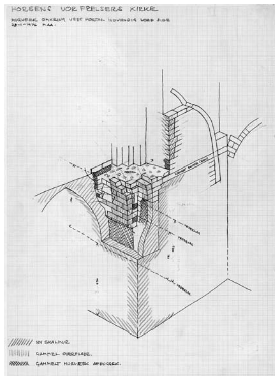
Fig. 221. Aksonometrisk skitse af murværk omkring vestportalens inderside mod nord (s. 5416, 5434). Tegnet af Morten Aaman Sørensen 1976. — Axonometric sketch of masonry around the inside of the west portal towards the north, 1976.
