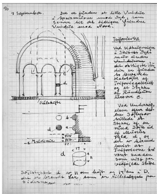
Fig. 53. Rester af triforium i søndre arkademurs østligste fag, jfr. fig. 50b. Skitse i Viggo Norns notebog (s. 90) fra restaureringen 1935-36. – Remains of triforium in the easternmost bay of the south arcade wall, cf. fig. 50b.
