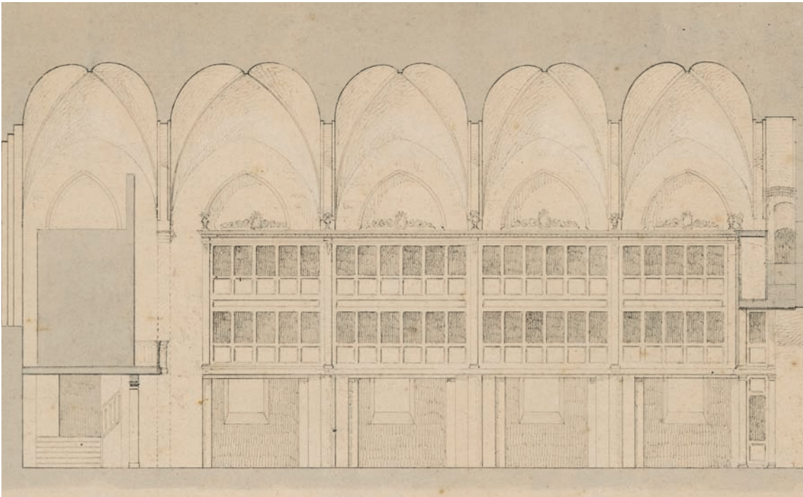
Fig. 158. Længdesnit i skibet mod nord med \dagger pulpiturer fra Kruuses og Hiernøes ombygning 1794-97 (s. 5542). 1:200. V. Th. Walther 1864 (jfr. fig. 20). I Horsens Museum. – Longitudinal section of the nave towards the north with \dagger pulpits made by Kruuse and Hiernøe 1794-97 (cf. fig. 20).
