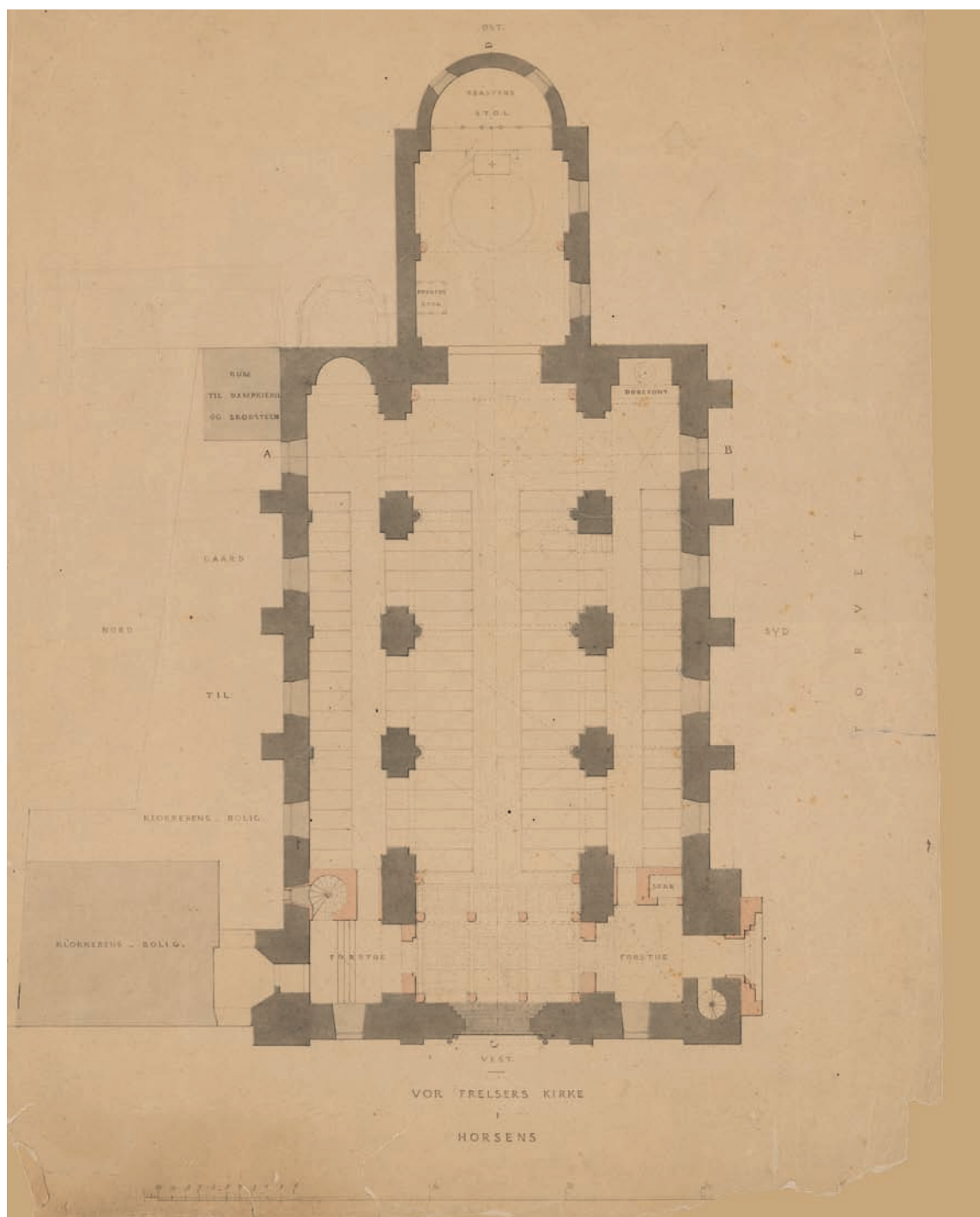
Fig. 21. Grundplan. Øst opad. 1:300. Restaureringsprojekt »A« ved V.Th. Walther 1864 (s. 5459). I Horsens Museum. – Ground plan. East at top. Restoration project 'A', 1864.
