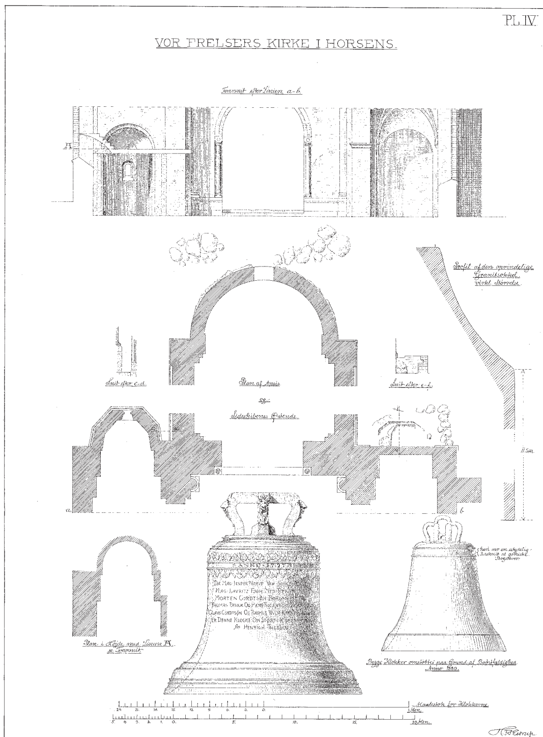
Fig. 27. Blad med grundplan af kor og triumfvæg samt diverse snit ved sidstnævnte. Endvidere sokkelprofil og to omstøbte \ddagger klokker nr. 1 og 8 (s. 5562, 5564). Plan og snit 1:200. Målt og tegnet af Hector Estrup 1884 på grundlag af skitser fra restaureringen 1879–81. – Page with ground plan of chancel and wall above chancel arch as well as various details of the latter. Also a base profile and two recast \ddagger bells, nos 1 and 8.
