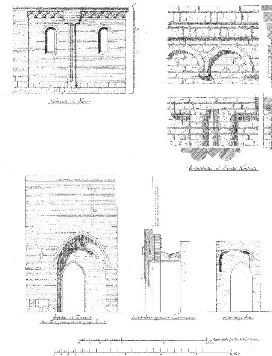
Fig. 26. Blad med facader, snit og detaljer af korets nordside og partiet omkring hovedindgangen mod Torvet efter fjernelsen af V.Th. Walthers portalindramning 1880. Facader og snit 1:200. Målt og tegnet af Hector Estrup 1884 på grundlag af skitser fra restaureringen 1879-81. — Page with facades, section and details of the north side of the chancel and the part around the main entrance towards the square after the removal of V.Th. Walther's portal frame in 1880.
