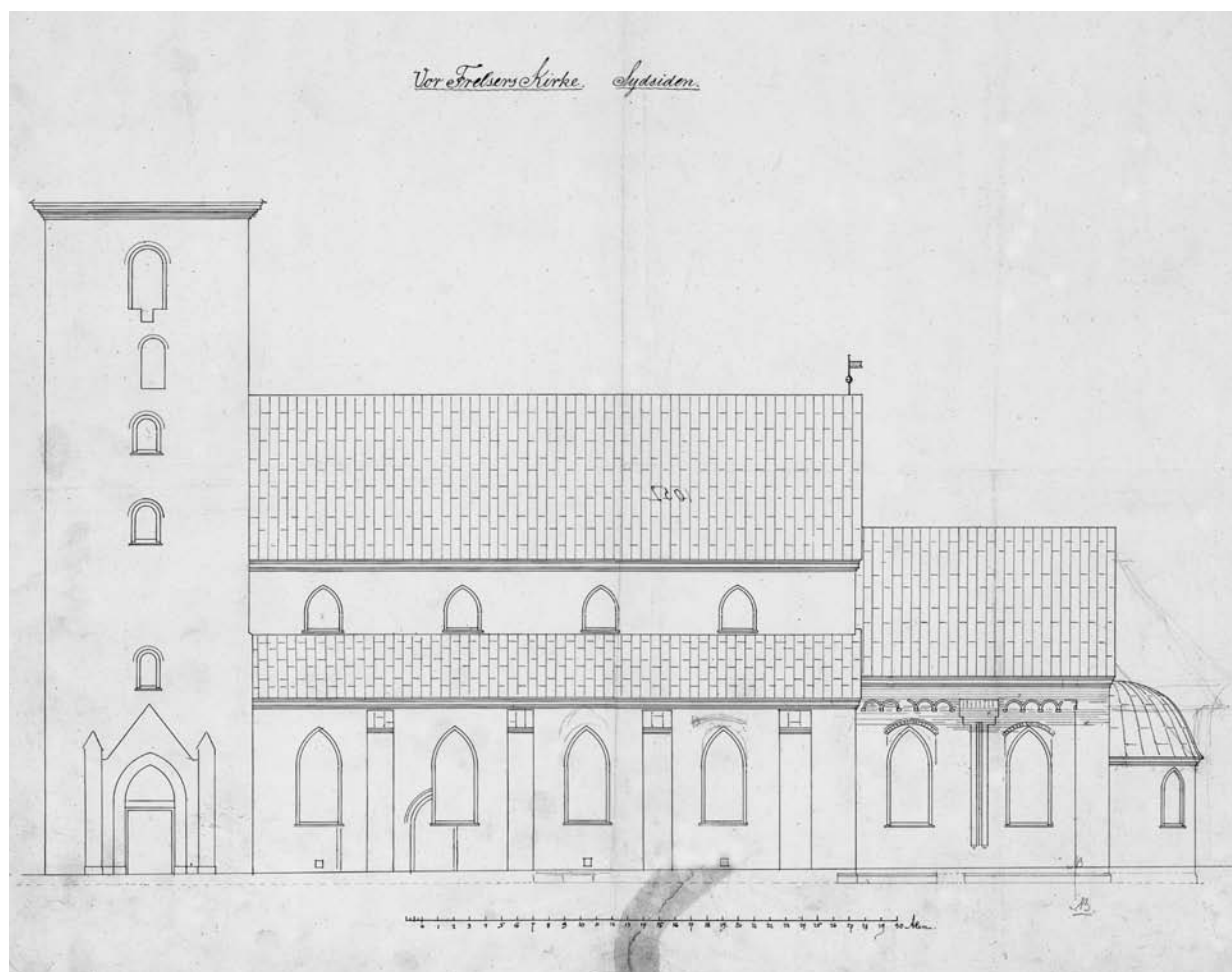
Fig. 36. Opstalt af kirkens sydside med angivelse af oprindelig sokkel og diverse murspor. Skitse ved Hector Estrup 1879. – Elevation of the south side of the church with indications of the original base and various traces of walls, 1879.
