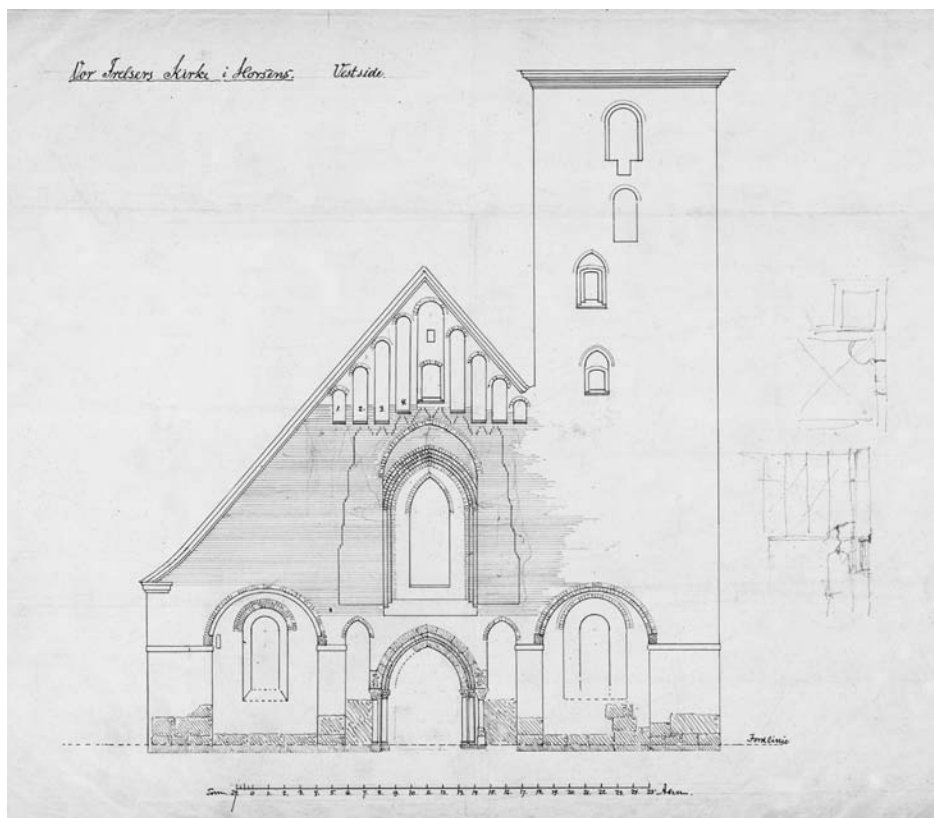
Fig. 38. Opstalt af kirkens vestfacade før restaureringen 1879-81. 1:300. Skitse ved Hector Estrup 1879. – Elevation of the west facade before the restoration of 1879-81.
