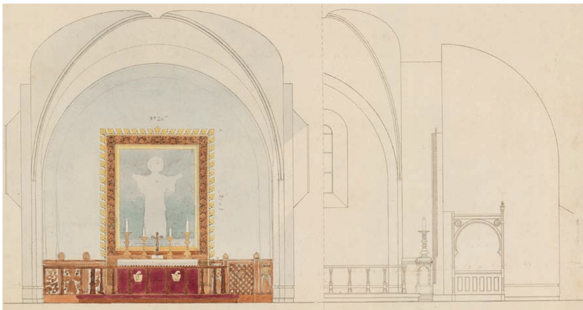
Fig. 101. Tvær- og længdesnit af korets østfag med altertavle, 1908, samt projekteret skriftestol (s. 5495, 5533). Tegning i Horsens Museum. – Cross- and longitudinal section of the easternmost bay of the chancel with altarpiece, 1908, and projected confessional.
