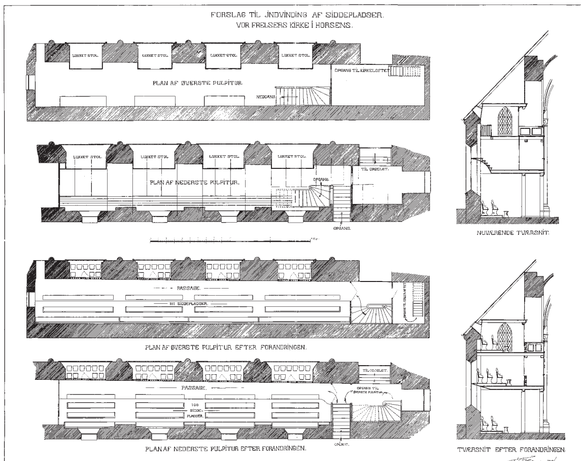
Fig. 160. Projekt til ændring af nordre sideskibs \dagger pulpiturer (s. 5545). 1:300. Tegnet af Hector Estrup 1886. I Horsens Museum. – Project for alteration of \dagger pulpits in the north aisle.
