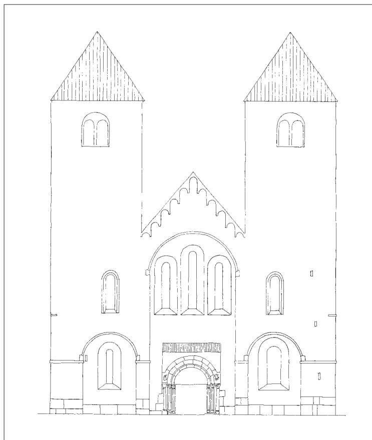
Fig. 42. Rekonstruktion af kirkens oprindelige vestfacade (s. 5411). 1:300. Tegnet af Mogens Vedsø 2004. – Reconstruction of the original west facade of the church.
