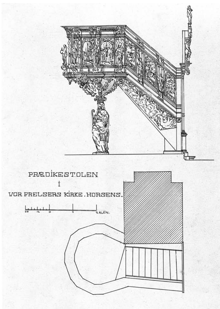
Fig. 129. Prædikestol 1670, jfr. fig. 125. 1:50. Plan og opstalt mod vest, tegnet af Thorvald Jørgensen 1886. Kunstakademiets Bibliotek. – Pulpit, 1670; cf. fig. 125. Plan and elevation towards west.
