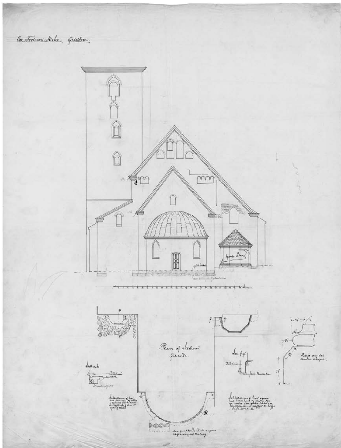
Fig. 34. Plan og opstalt af kirkens østende med angivelse af diverse fundamenter og murspor. Skitse ved Hector Estrup 1879. 1:300. — Plan and elevation of the east end of the church with indications of various foundations and traces of walls.
