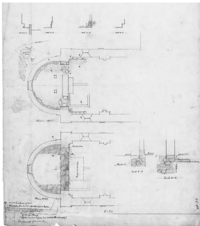
Fig. 47. Plan og diverse snit i korets østende. Syd opad. 1:300. Målt og tegnet af Viggo Norn 1935 og 1949. I Horsens Museum. – Plan and various sections of the east end of the chancel. South at top.
