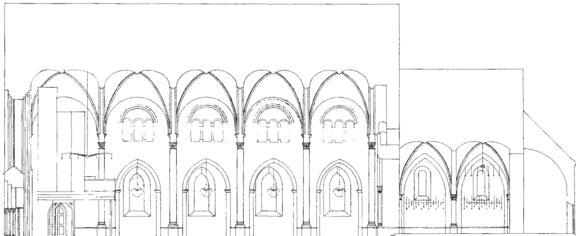
Fig. 167. Belysningsprojekt for kirken 1979 (s. 5554). Tegning af Inger og Johannes Exner. Ved embedet. – Lighting project for the church, 1979, by Inger and Johannes Exner.
