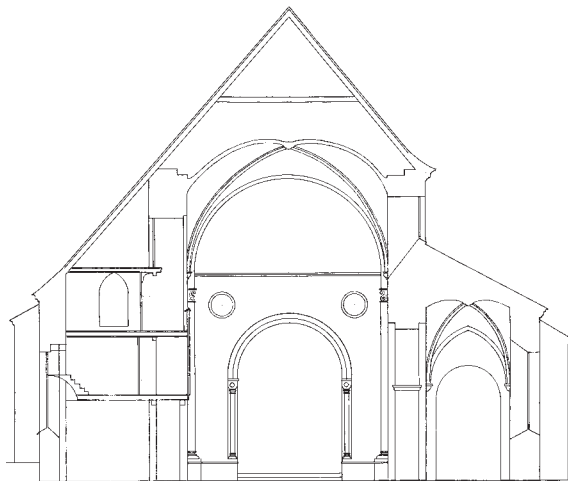
Fig. 82. Tværsnit i skibet mod øst. 1:300. Målt og tegnet af Viggo Norn 1935 forud for restaureringen. I Horsens Museum. – Cross-section of the nave towards the east, 1935, before the restoration.
