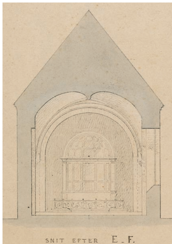
Fig. 104. Tværsnit i koret mod øst med alterudsmykning fra Kruuses og Hiernøes ombygning 1794-97 (s. 5496). 1:150. V.Th. Walther 1864 (jfr. fig. 20). I Horsens Museum. – Cross-section of the chancel towards the east with altar decoration made by Kruuse and Hiernø 1794-97 (cf. fig. 20).
