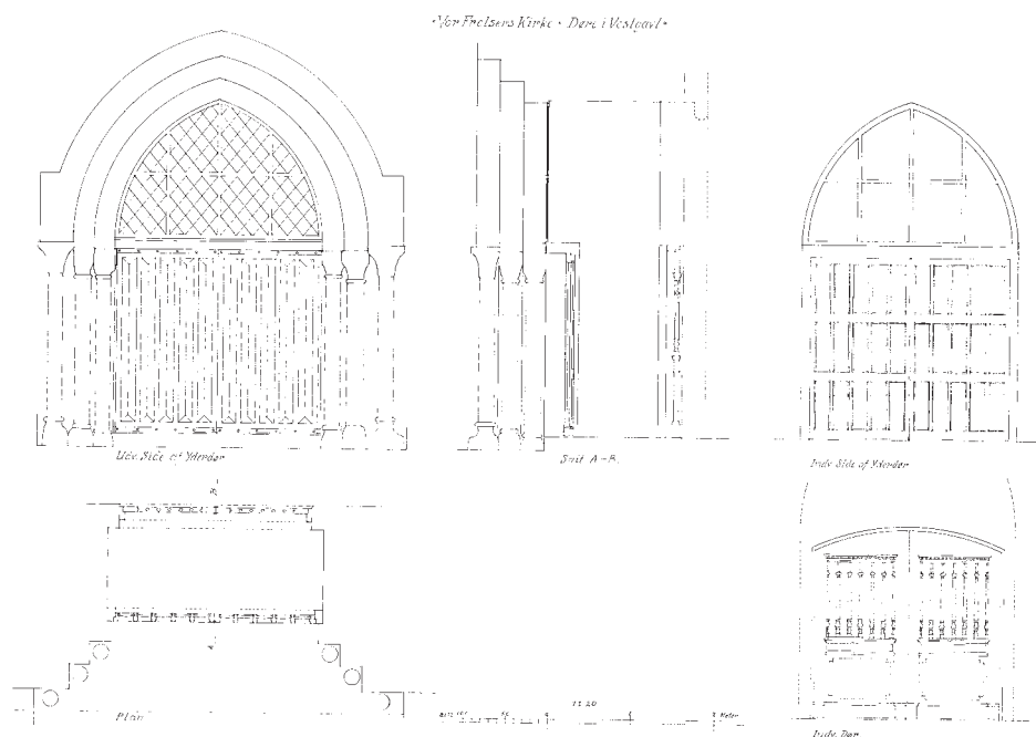
Fig. 155. Dørføj nr. 2, 1935-36 og †dørføj nr. 3, 1873(?), omdannet 1935-36 (s. 5539). Tegning af Viggo Norn. 1:100. I Horsens Museum. – Door no. 2, 1935-36 and †door no. 3, 1873(?), reconstructed 1935-36. Drawing by Viggo Norn.
