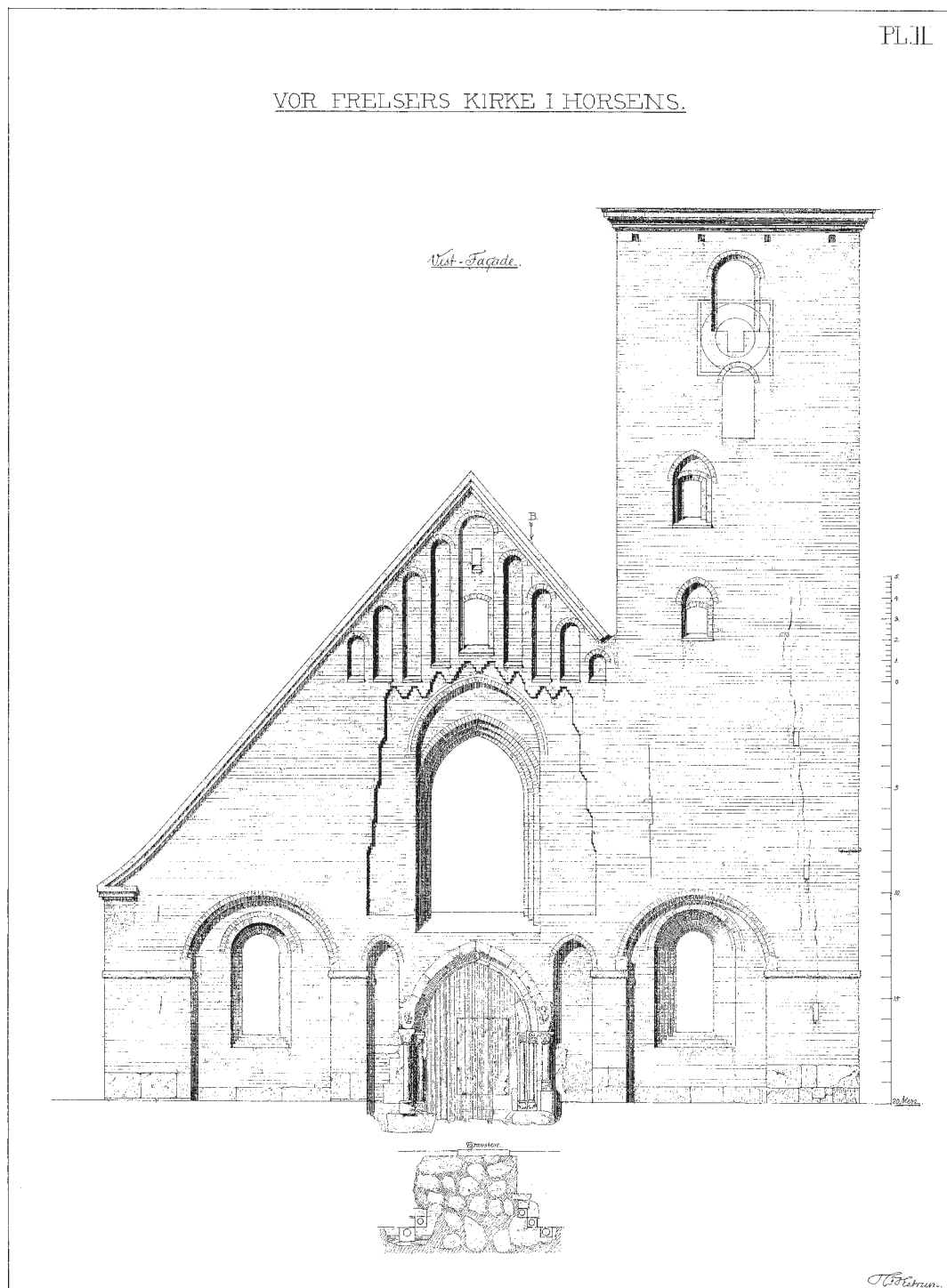
Fig. 25. Blad med vestfacade før restaureringen 1879-81; dog er vinduerne vist i den restaurerede skikkelse og portalen efter fjernelsen af \ddagger kalkhus, jfr. fig. 218. 1:200. Målt og tegnet af Hector Estrup 1884 på grundlag af skitser fra restaureringen. – Page with west facade before the restoration of 1879-81; however, the windows are shown in the restored form and the portal after the removal of the \ddagger chalk house, cf. fig. 218.
