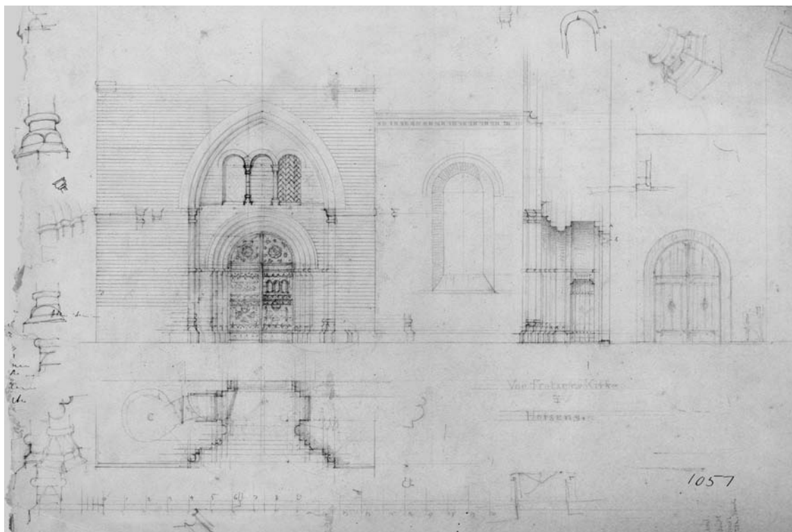
Fig. 78. Indgangsportalen mod Torvet (s. 5466). Udkast ved H. B. Storck 1880. – Entrance portal towards the square Torvet. Draft 1880.
