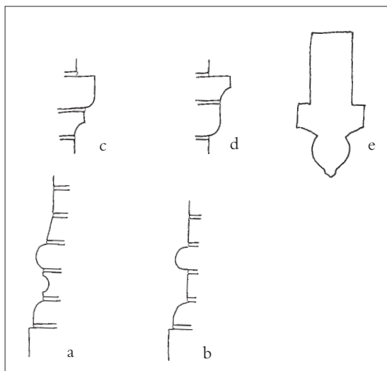
Fig. 51. Profiler og detaljer. 1:20 (a-d) og 1:10 (e). a. Arkadepillernes sokkel (s. 5424). b. Hvælvpillernes sokkel i midtskibet (s. 5424). c. Kragbånd i søndre arkaderække; hhv. østre arkades østre og vestre arkades vestre kragbånd (s. 5424). d. Øvrige kragbånd i søndre arkaderække (s. 5424). e. Hvælvrække benyttet i såvel koret som midt- og sideskibe (s. 5441). Tegnet af Mogens Vedso 2004 efter opmålinger ved Viggo Norn 1935-36. – Profiles and details. 1:20 (a-d) and 1:10 (e). a. Base of arcade pillars. b. Base of arch pillars in nave. c. Cordons in south arcade row; the eastern cordon of the east arcade and the western cordon of the west arcade respectively. d. The other cordons in southern arcade row. e. Vault rib used in chancel as well as nave and side aisles. Drawn by Mogens Vedso in 2004 after measurements by Viggo Norn in 1935-36.
