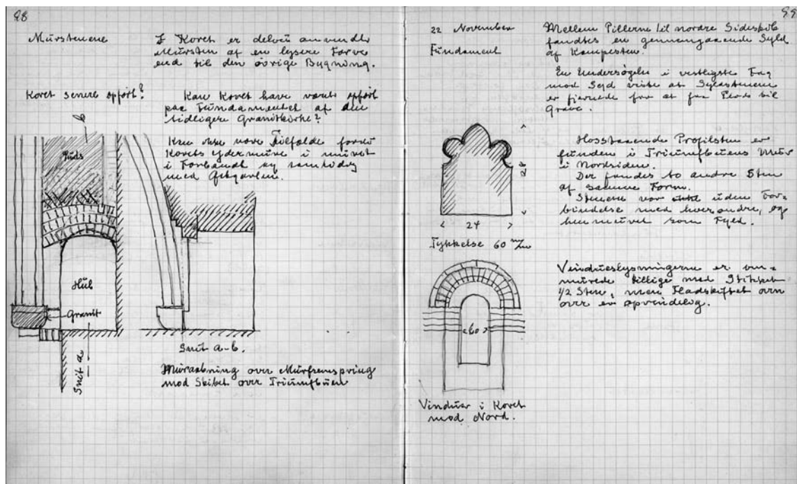
Fig. 49. Detaljer af gang over korbuen med dør til nordre arkademurs triforiegalleri (s. 5423) samt ribbesten (s. 5437), fundet i triumfmurens niche, og detalje af korets nordvestlige vindue (s. 5417). Skitser i Viggo Norns notebog (s. 96-97) fra restaureringen 1935-36. — Details of passage over chancel arch with door to the triforium gallery of the north arcade wall and ribbing brick, found in the niche of the wall above the chancel arch, and detail of the north west window of the chancel.
