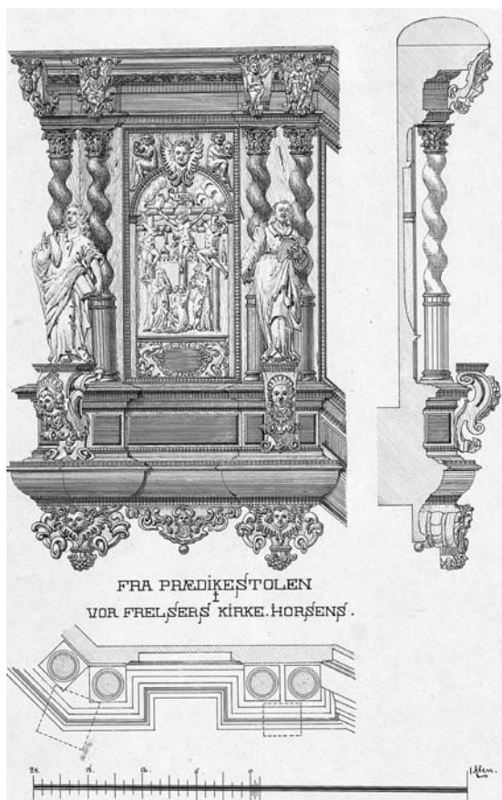
Fig. 128. Arkadefag af prædikestol 1670, jfr. fig. 125 (s. 5516). 1:20. Plan, opstalt og snit, tegnet af Thorvald Jørgensen 1886. Kunstakademiets Bibliotek. – Arcade bay of pulpit, 1670; cf. fig. 125. Plan, elevation and section.
