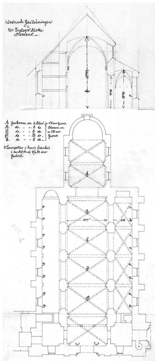
Fig. 232. Grundplan med angivelse af placeringen af kirkens fem lysekroner og 18 væglampetter, 1889 (s. 5554). Tegning ved Hector Estrup. I Horsens Museum. – Ground plan with indications of the placing of the church's five chandeliers and 18 wall lampettes, 1889.
