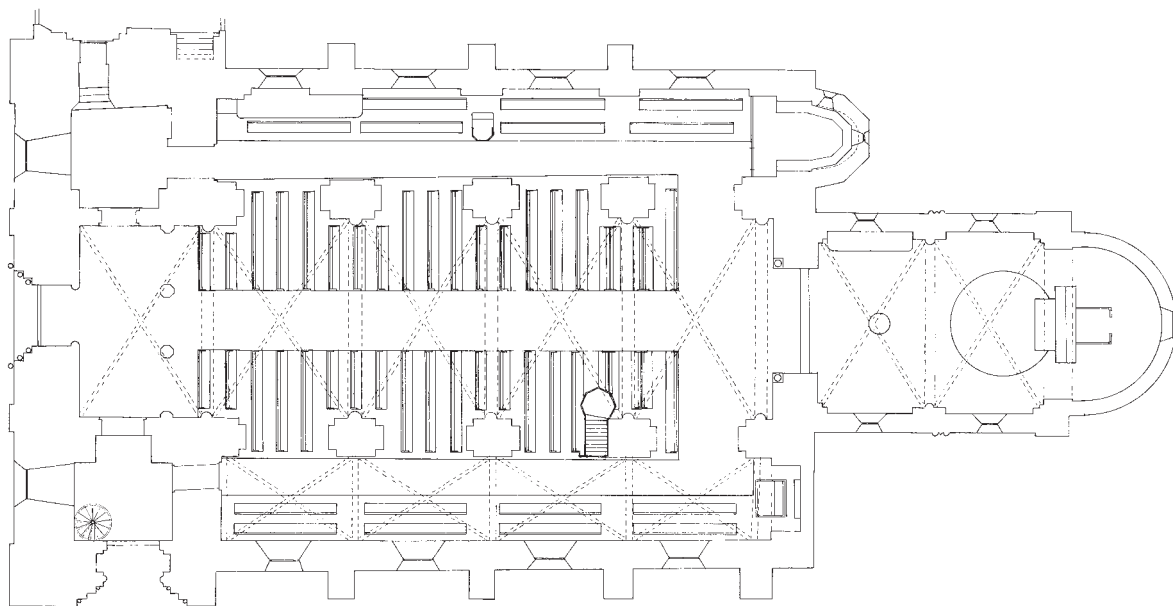
Fig. 85. Grundplan. 1:300. Målt og tegnet af Viggo Norn 1935 forud for restaureringen. I Horsens Museum. – Ground plan, 1935, before the restoration.
