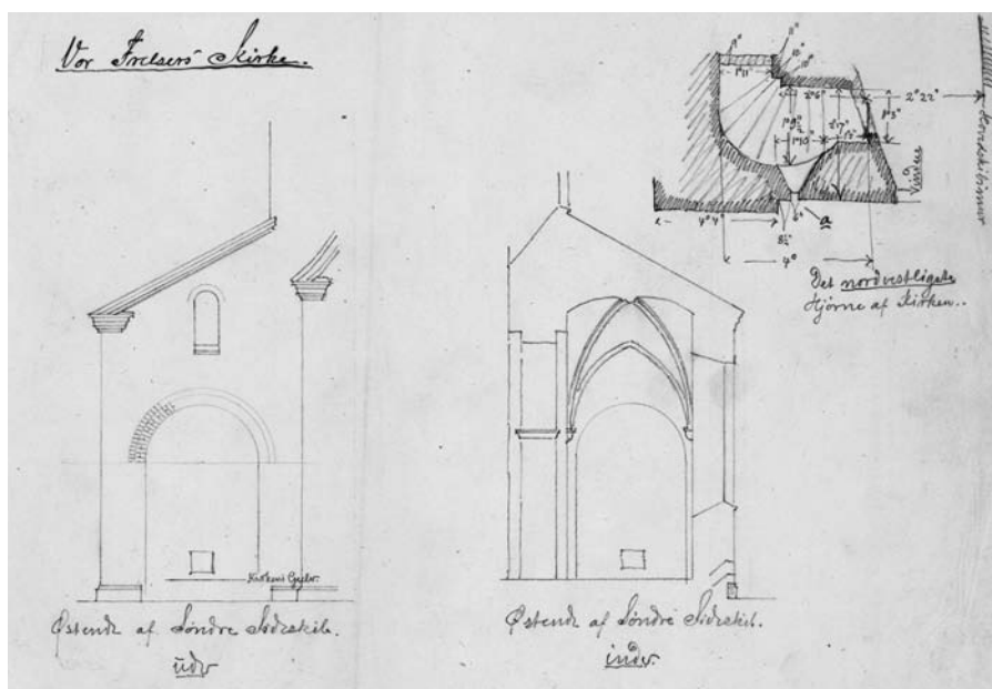
Fig. 37. Østenden af søndre sideskib (s. 5409) samt plan af nordre tårntrappes nedre del, jfr. fig. 64 (s. 5436). Skitse fra Hector Estrups bygningsundersøgelse 1879. – Eastern end of south side aisle and plan of the northern tower stairs, cf. fig. 64. Sketch from Hector Estrup's building survey, 1879.
