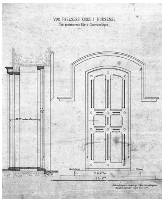
Fig. 157. †Dørfloj nr. 4, 1873–74, udført efter tegning af V.Th. Walther (s. 5540). I Horsens Museum. – †Door no. 4, 1873–74. Drawing by V.Th. Walther.
