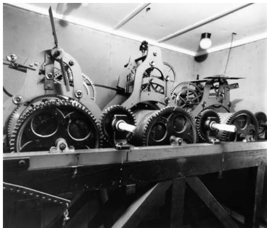
Fig. 175. Tårnure nr. 1, 1881, udført af urmager J. Chr. Jensen, Bornholm (s. 5558). Roberto Fortuna fot. 2004. – Tower clock no. 1, 1881, by clockmaker J. Chr. Jensen, Bornholm.
