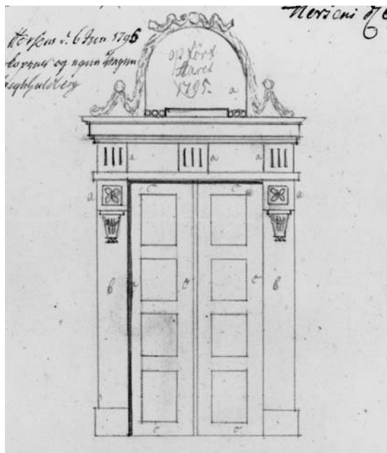
Fig. 7. Tegning til portal (nr. 2) ved Jens Hiernøe 1795 (s. 6064). a angiver sandsten, b mursten og c dørfløjene af egetræ fra den tidligere dør. – Drawing for portal (no. 2) by Jens Hiernøe, 1795. a is sandstone, b brick and c the oak panels from the former door.
