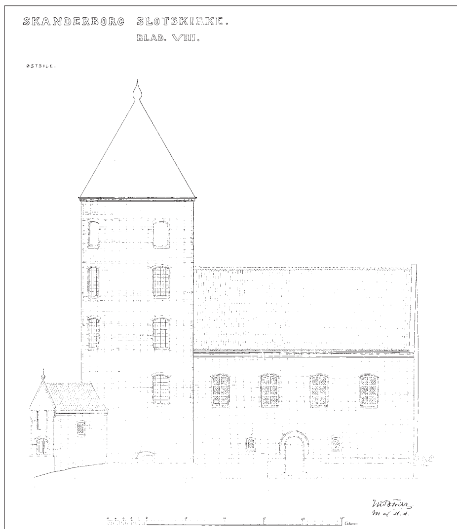
Fig. 24a. Opstalt af østfacaden. Tegnet af M. B. Fritz 1909. – Elevation of the east facade.
