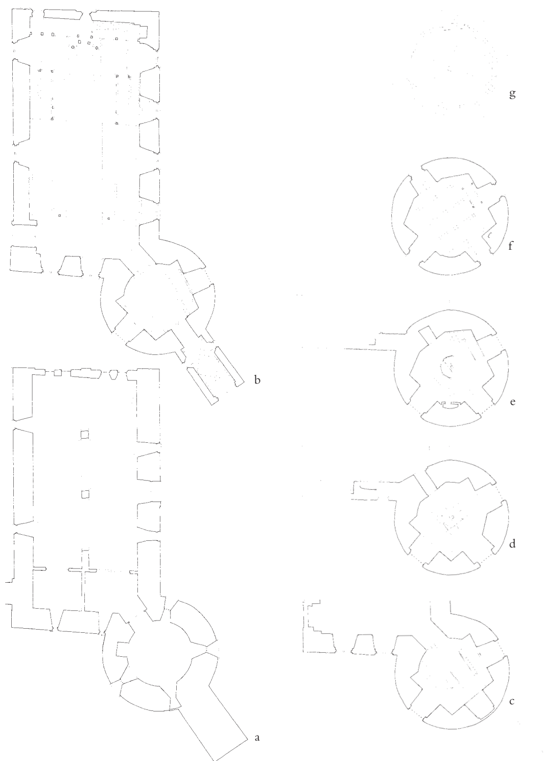
Fig. 18a-g. Planer. 1:300. Målt og tegnet af Peter Kristiansen 1988. a. Kælderen. b. 1. stokværk. c-f. Tårnets pulpituretage samt 2.-4. stokværk. g. Spiret. — Plans. a. Basement. b. 1st floor. c-f. Gallery level and 2nd-4th floor of the tower. g. Spire.
