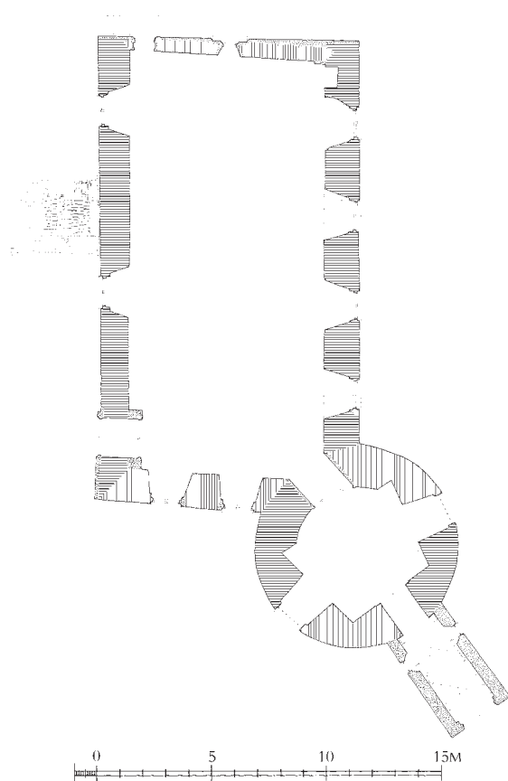
Fig. 15. Grundplan. 1:300. Nord opad. Målt og tegnet af Peter Kristiansen 1988, kældertrappe tilføjet efter opmåling 1979 i Skanderborg Museum; redigeret af Mogens Vedsø 2006 (sml. fig. 18b). – Ground plan. North at top.
