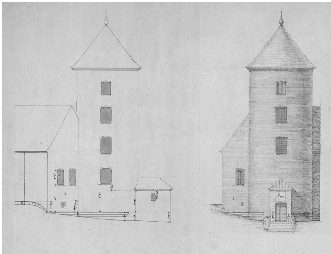
Fig. 22a. Opstalter af tårnet set fra sydvest og sydøst. Tegnet af V. Th. Walther 1878. – Elevations of the tower viewed from the south west and the south east.
