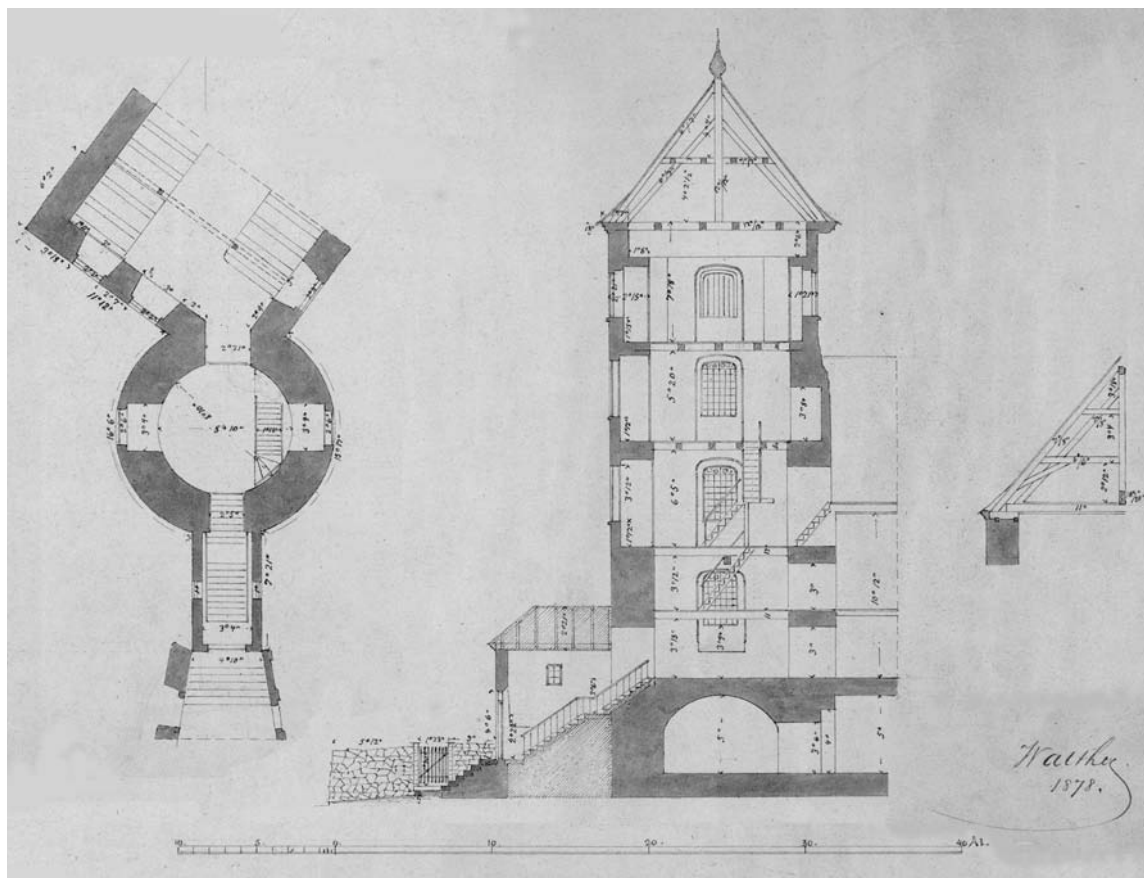
Fig. 22b. Plan og tværsnit af tårnet samt udsnit af kirkens tagværk (th.). Tegnet af V.Th. Walther 1878. – Plan and section of the tower and section of church roofing.
