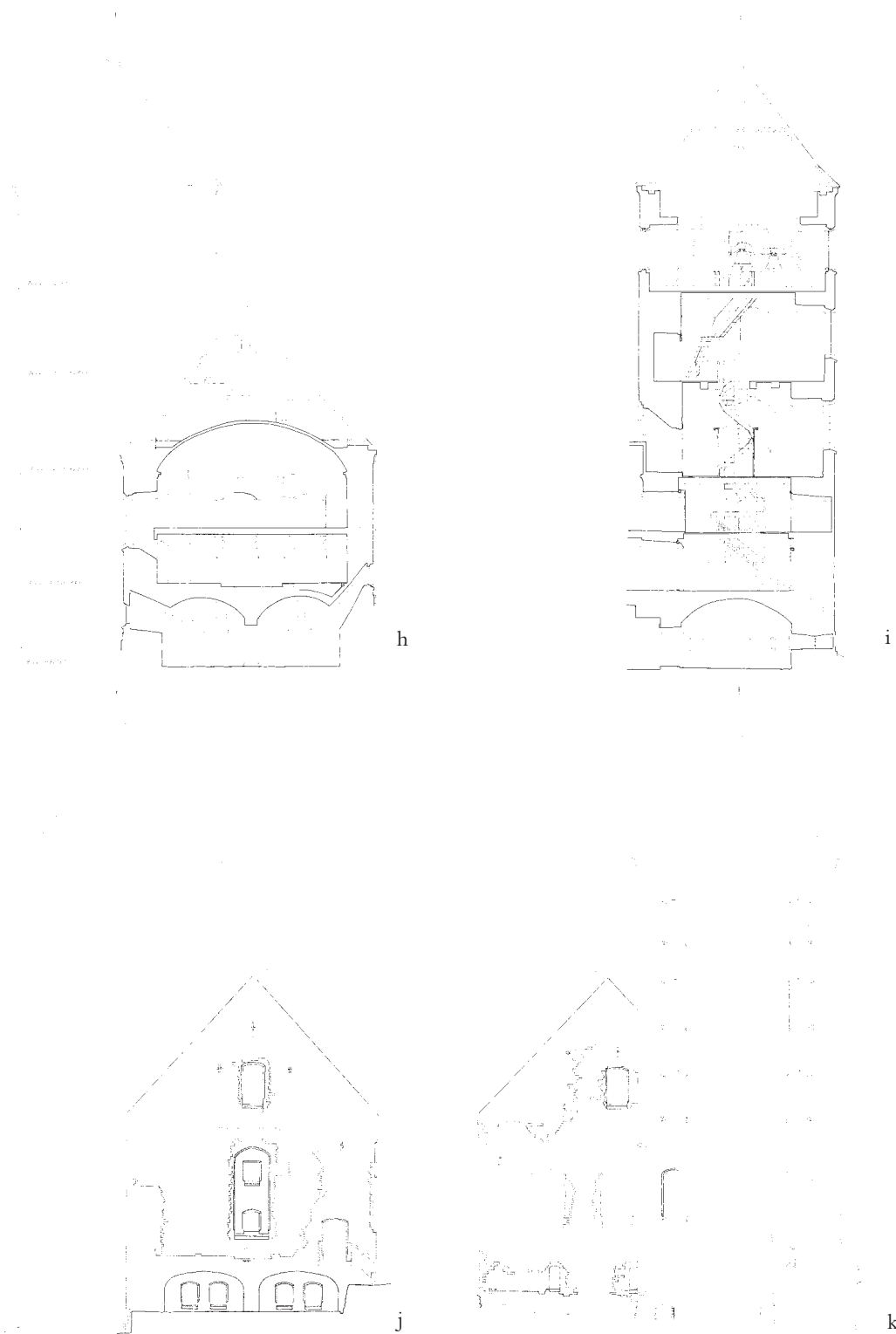
Fig. 18h-k. Snit og opstalter. 1:300. Målt og tegnet af Peter Kristiansen 1988. h. Tværsnit set mod syd. i. Tværsnit gennem tårnet set mod nordøst. j. Nordfacaden. k. Sydfacaden. — Sections and elevations. h. Section viewed towards the south. i. Section through the tower viewed towards the north east. j. Elevation of the north facade. k. Elevation of the south facade.
