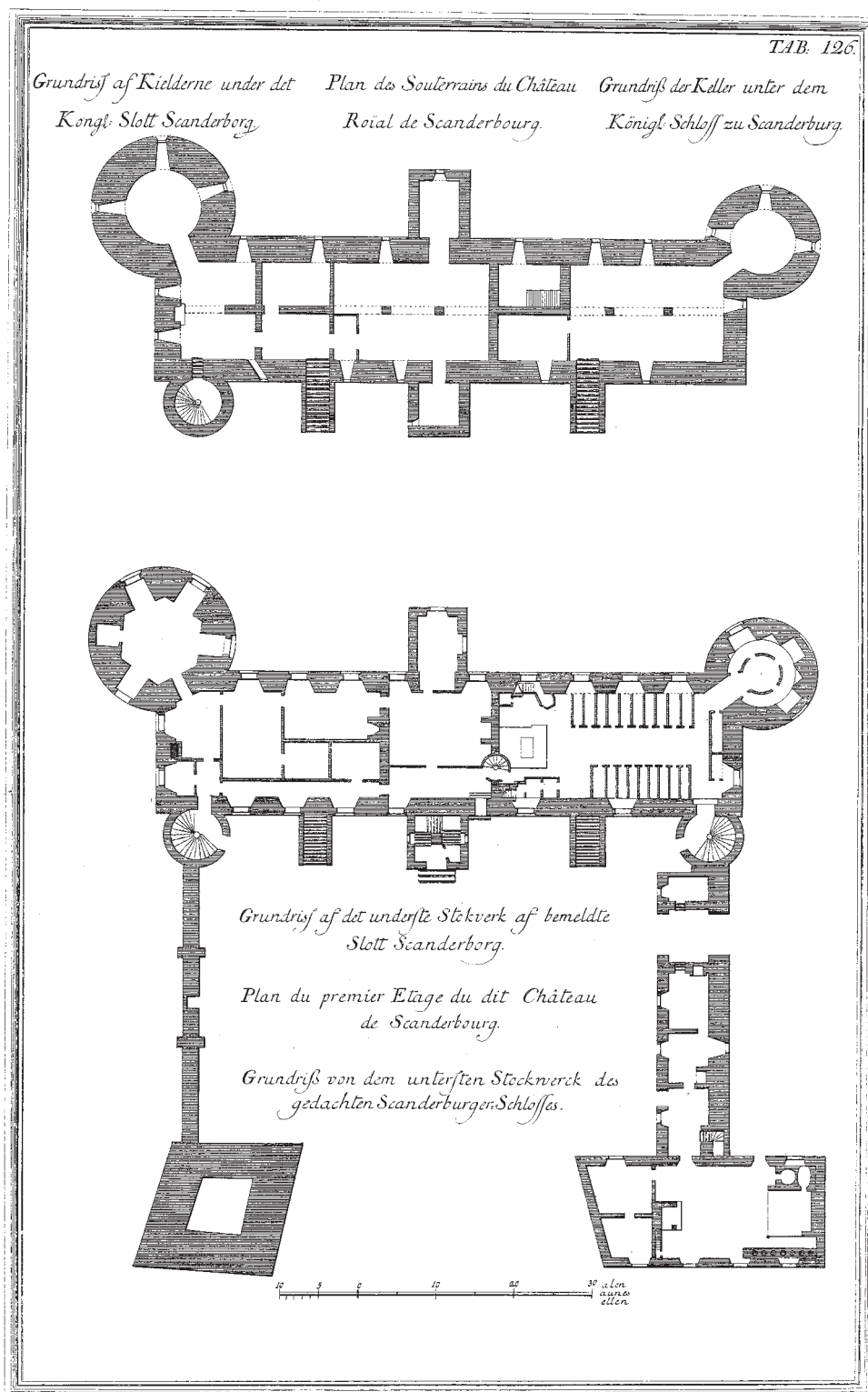
Fig. 11. Planer af Skanderborg Slots kælder og 1. stokværk. Efter Lauritz de Thura: Den danske Vitruvius , II, 1749. – Plans of basement and first floor of Skanderborg Castle.
