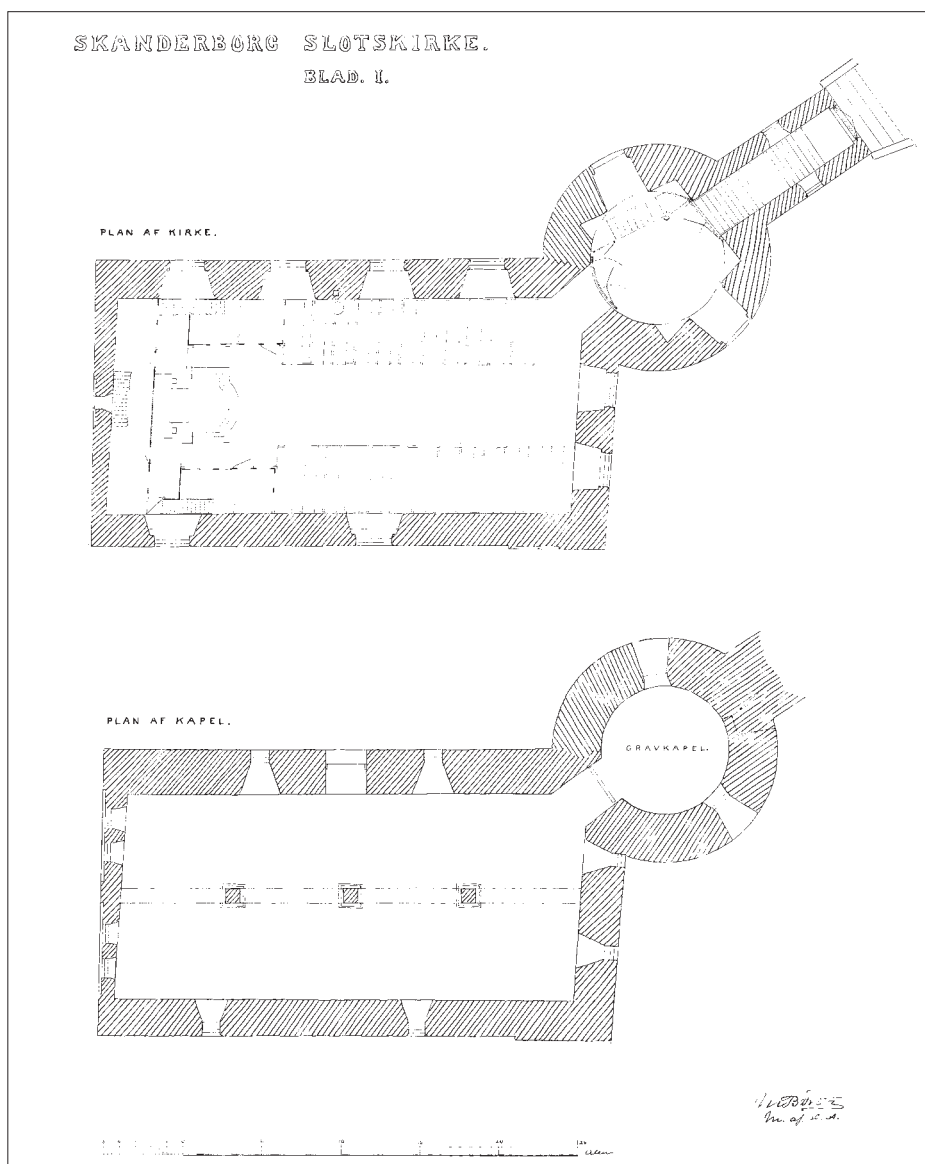
Fig. 24b-c. Planer af kirken og kælderens. Tegnet af M. B. Fritz 1909. – Plans of the church and the basement.
