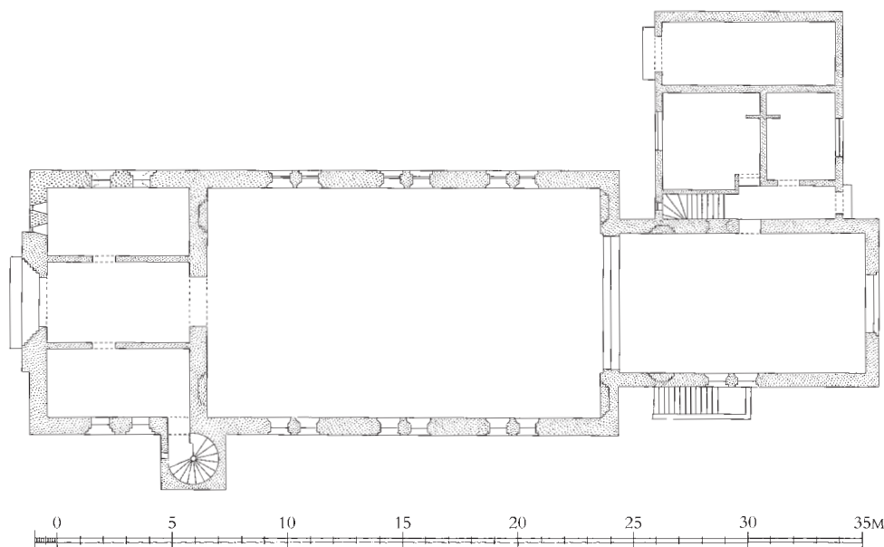
Fig. 3. Grundplan. 1:300. Tegnet af MN 2006 efter Steensen & Varming, Århus 1972. – Ground plan.
