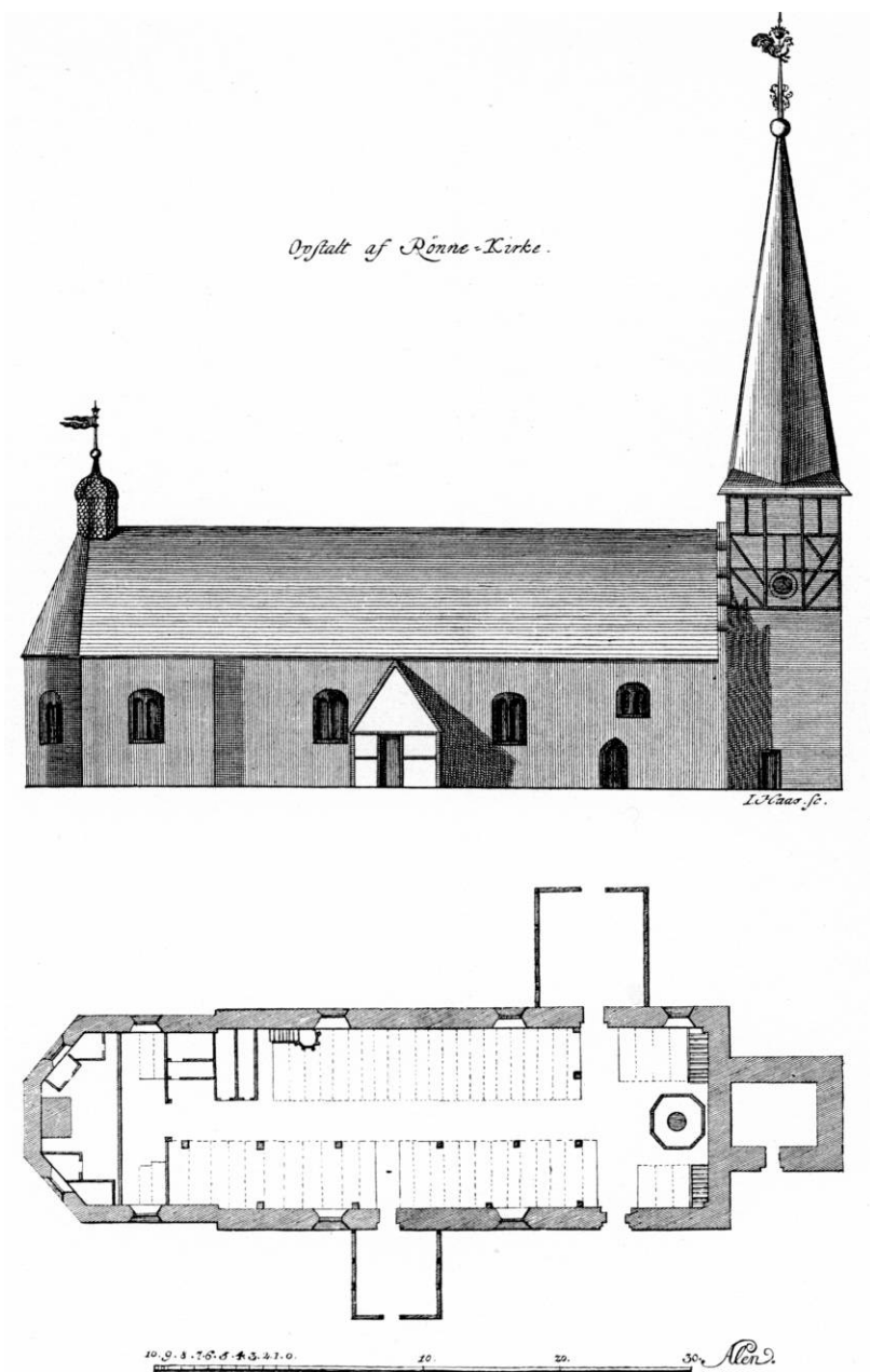
Fig. 6. Rønne kirke, plan og opstalt af nordsiden (vest til højre) efter Thurah. Opmålingen, som muligvis er udført kort efter 1757 (sml. våbenhus, s. 46) og i hvert tilfælde før 1759 (Thurahs dødsår), giver et i hovedtrækkene pålideligt billede af kirken indtil ombygningen 1797.
