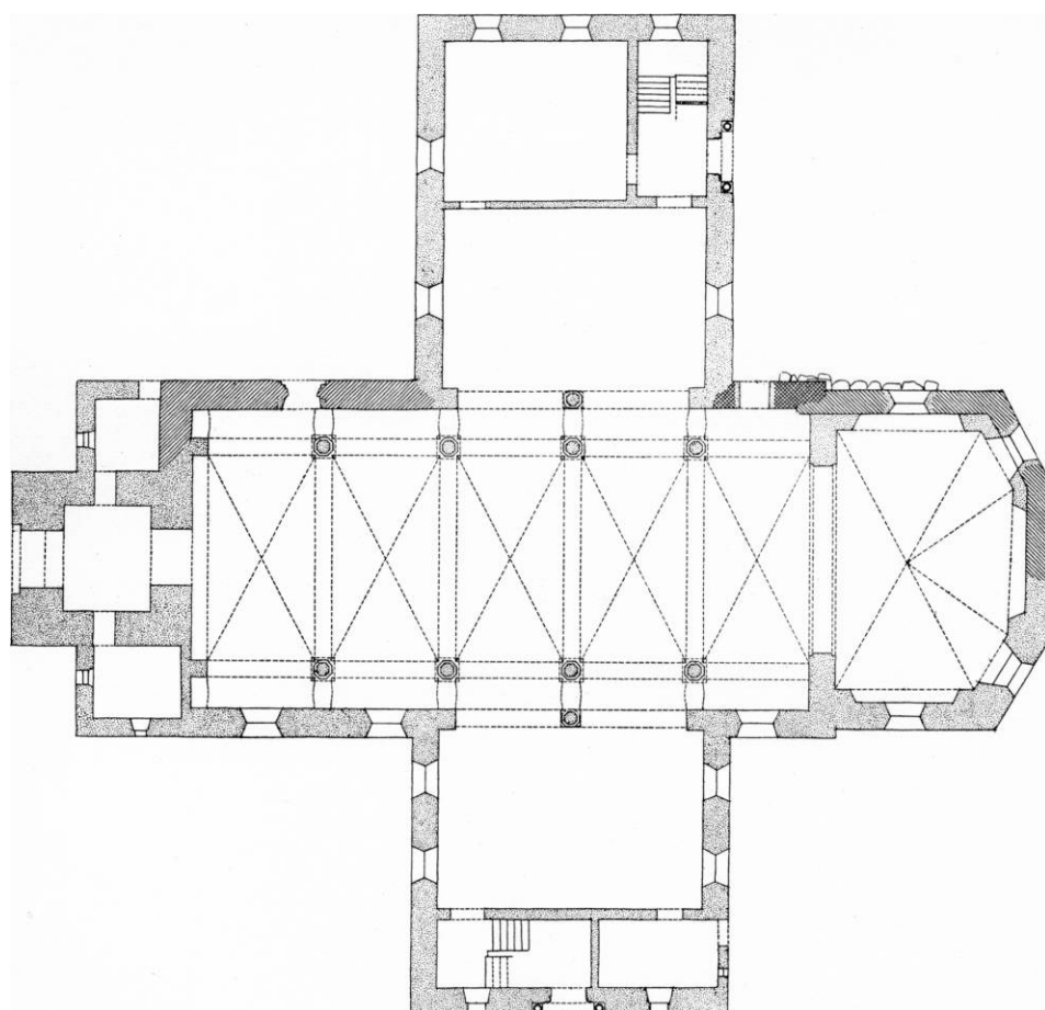
Fig. 3. Rønne kirke, nuværende plan, 1:300. Målt af C. G. S. 1952.
