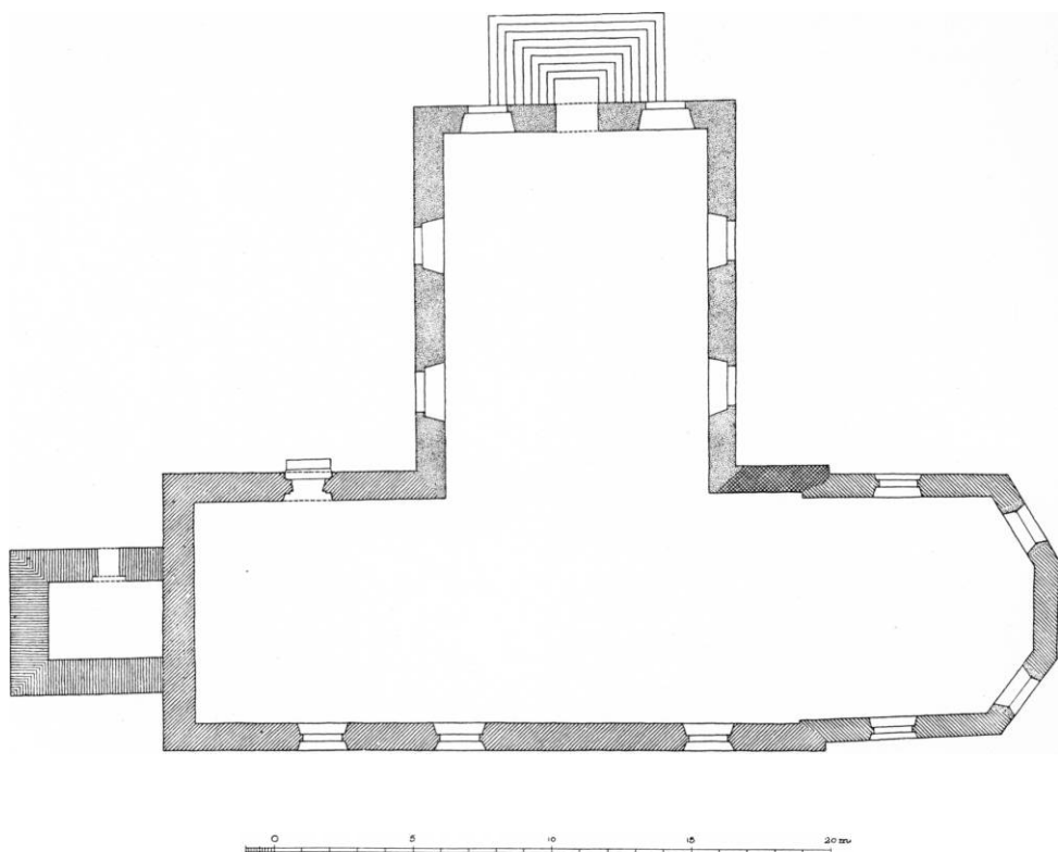
Fig. 4. Rønne kirke før ombygningen. Plan, 1:300. Efter opmåling af arkitekt H. Chr. M. Steen (Tove Bojesen 1953).
