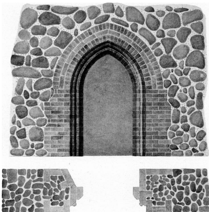
Fig. 7. Rønne kirke, †syddør (ca. 1:50), målt 1916 af Carl H. Nimb.
