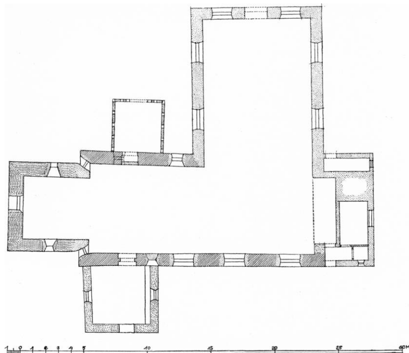
Fig. 2. Neksø. Plan. 1:300. Efter opmåling af Charles Christensen 1939.
