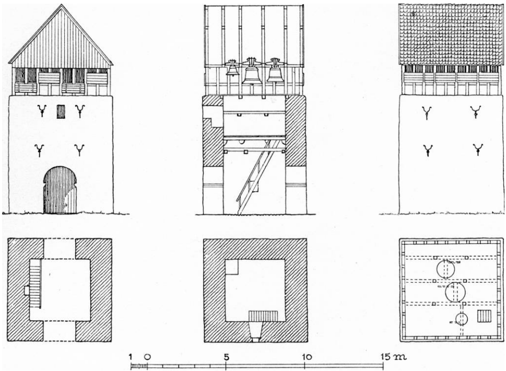
Fig. 4. Å kirke. Planer, snit og opstalter af det i 1874 nedbrudte klokketårn. Mål 1:250. Efter forarbejde af E. Blichfeldt til tegningen i B.æ.K., pl. 34 6 .
