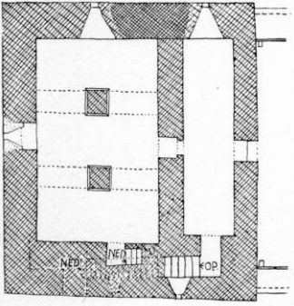
Fig. 3. Å kirke. Planer i 1:300, målt af Charles Christensen 1938. Nederst grundplan af hele kirken, derover planer af 2. og 3. tårnetage. De i 1874 nedbrudte lang- og tværarkader i skibet er indpunkterede efter opmålingerne i B.æ. K. Delelinjerne i tværskillerummets midtpille og i langskillerummets østligste pille angiver grænserne for to senere udhugninger, som var foretaget på de nævnte pillers østsider for at skaffe bedre pladsforhold.
