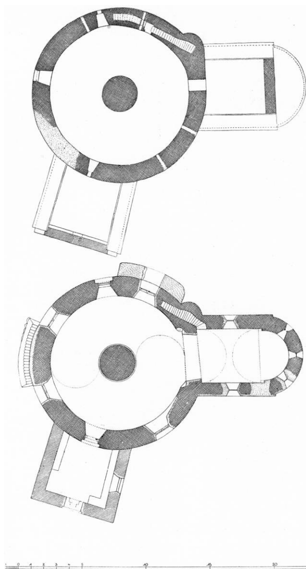
Fig. 4. Nykirke. Grundplaner. Mål 1:300. Over-stokværket øverst. Målt af Charles Christensen 1939.
