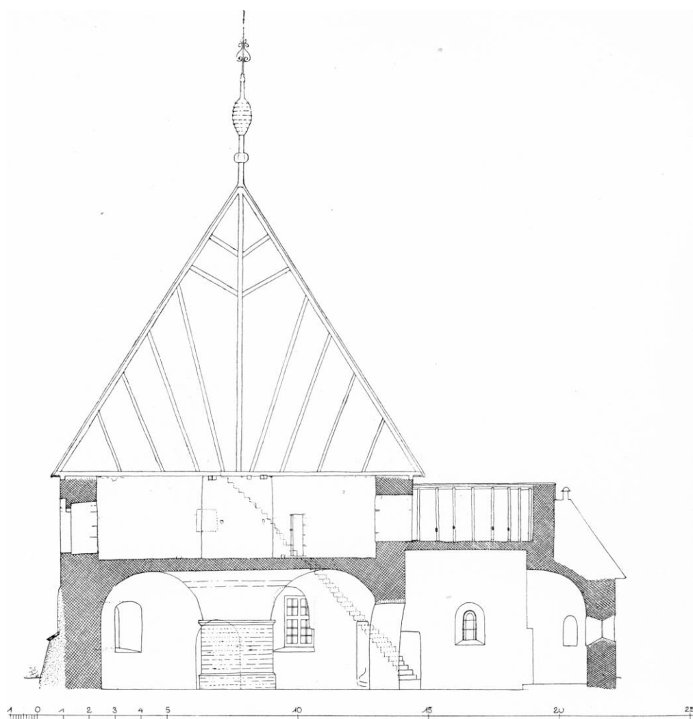
Fig. 5. Nykirke. Langsnit, set mod nord (1:200). Målt af Charles Christensen 1939.
