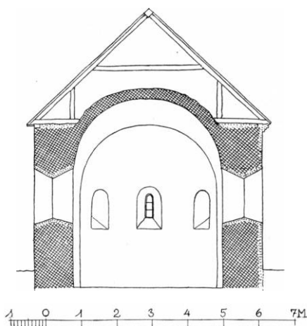
Fig. 8. Nykirke. Tværnsnit af koret set mod øst. Målt af Charles Christensen 1939.
