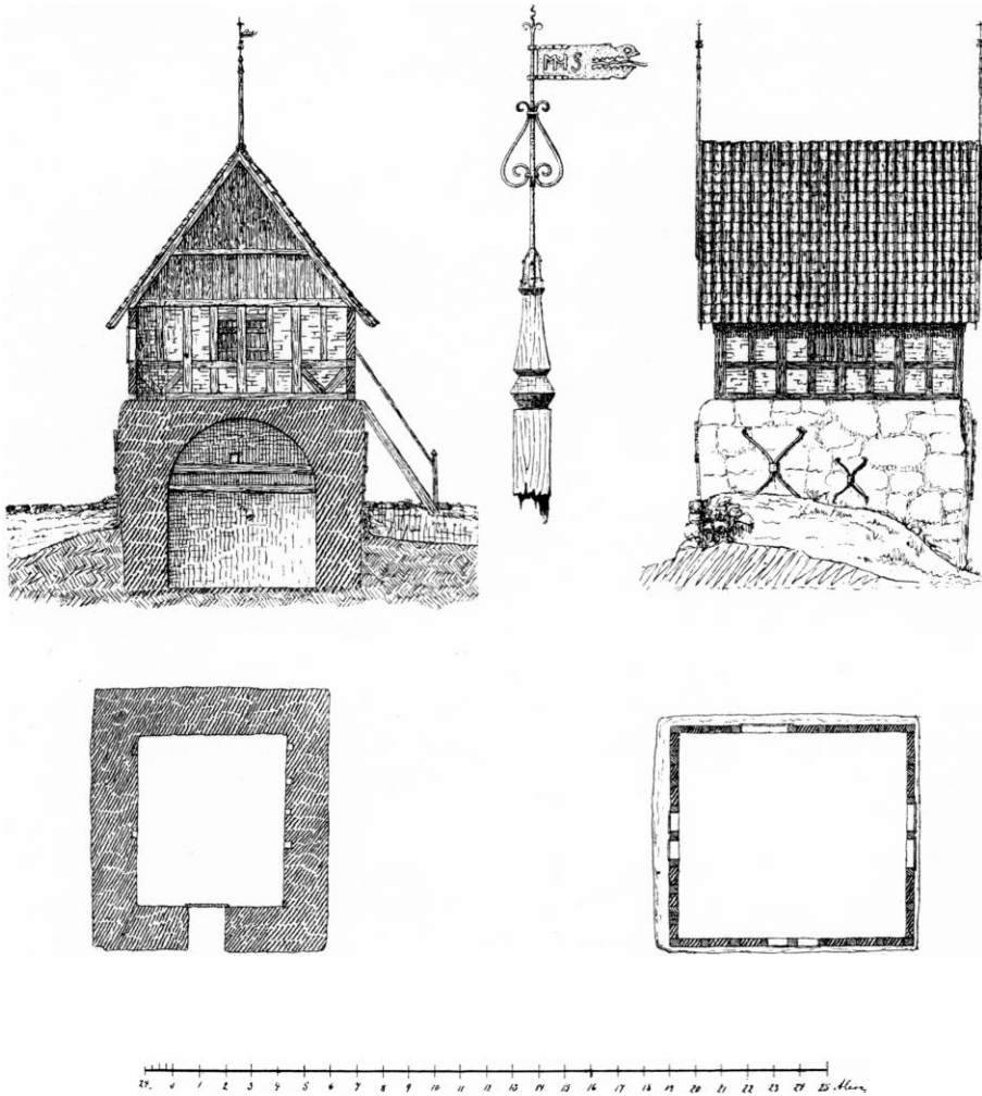
Fig. 2. Ruts kirke. Klokketårn. Øverst snit, set mod vest, sydfaçade og i midten en husbrand, nederst planer af de to stokværk. Målt af M. Bidstrup 1887.
