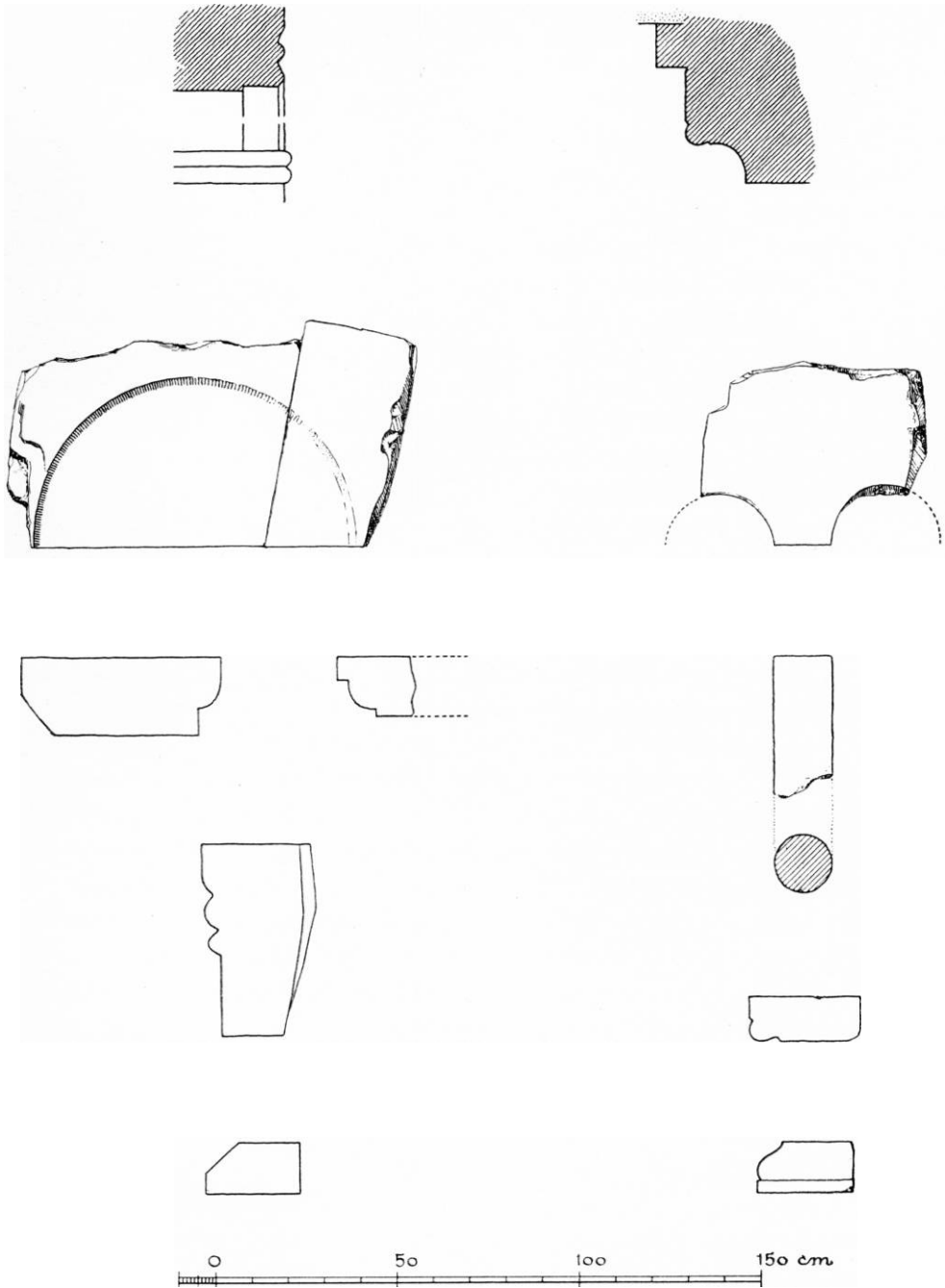
Fig. 8. Ruts kirke. Øverst t.v. kragbånd og snit af stik fra \uparrow våbenhusportal (efter skitse af H. J. Holm, notesbog F, s. 34, Kunstakad. bibl.), t.h. snit gennem sydportalens østkarm. Derunder t.v. tympanon og konsoller fra \uparrow vestportal, portalkonsol fra \uparrow våbenhus samt sokkelsten, vistnok sammesteds fra, t.h. overligger og søjlestump fra sydvindue i \uparrow tårnets 2. etage, kragsten af ukendt proveniens samt sokkelsten fra \uparrow vesttårnet. Alt til venstre er af silurkalk, til højre af frådsten. Mål 1:20. C. G. S. 1956.
