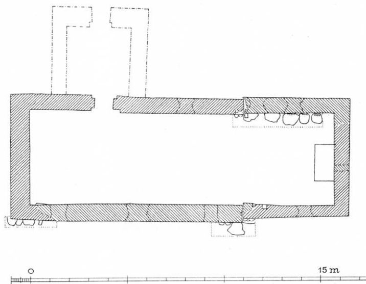
Fig. 3. Gudhjem. Plan (C. G. S. 1957) og opstalt (laveret blyantstegning af Andreas Clemmensen 1893). 1:200. På planen, som er en opmåling af den nuværende ruin, er vinduesstederne og våbenhuset indpunktet efter Clemmensens og Kornerups opmålinger.
