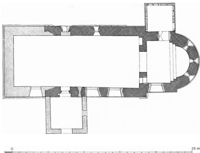
Fig. 3. S. Povls kirke. Plan 1:300, målt af G. G. S. 1957.
