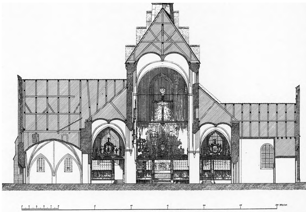
Fig. 15. S. Olai kirke. Tværsnit, set mod øst. 1:300. Tegnet af Christen Larsen 1901 til Ældre nord. Arch. 4. serie, 2. rk., her, som ved de følgende opmålinger fra 1901, reproduceret efter originaltegningerne i Nationalmuseet.
