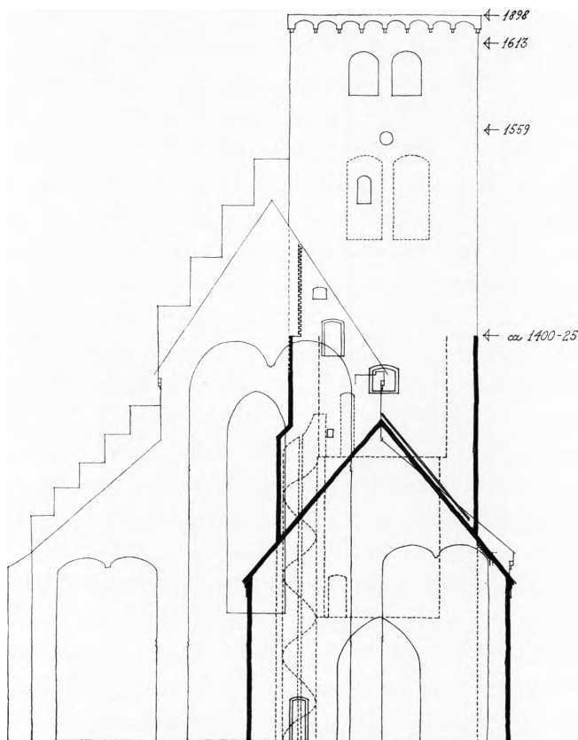
Fig. 11. S. Olai kirke. Tværsnit og tårn. Målskitse 1:300. Tegnet af K. de F. L. Den kraftigt optrukne kontur viser dels den enskibede kirke, dels tårnets ældste del; forløbet af den med tårnet samtidige spindeltrappe og hertil hørende døre er kun delvis kendt (p. 57, 61, 103, 105, 108).
