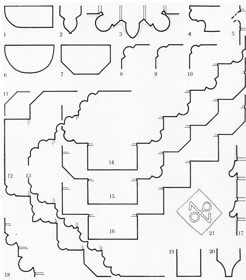
Fig. 22. S. Olai kirke. Profiler. 1:10. Tegnet af El. M. Tårn: 1. Vestportalens bueslag. 2. Hvælvingsribbe. Oxes kapel : 3. Hvælvingspille sammensat af ribbeprofil og de to rundstave, som markerer kappernes fødselslinier; den sidste findes også i dørens bueslag. 4. Fra fladbuet stik i trappens overdækning. 5. Vandnæseprofil, delvis rekonstruktion. Det treskibede langhus : 6—7. Væg- og arkadepillernes halvrunde og affasede buevederlag. 8—10. Væg- og arkadepillernes hjørnerundstave (i kronologisk rækkefølge). 11. Affaset hjørneled fra arkadepillernes opgående del. 12. Karmprofil fra syddøren. 13. Karmprofil fra søndre sideskibsmurs østligste vindue. 14—15. Profil fra østafsnittets arkadebuer i henholdsvis syd og nord. 16. Arkadebue i vestafsnittet. 17. Vederlagsbånd på væg- og arkadepiller. 18. Buefrisekonsol fra østafsnittets nordside. 19. Ribbeprofil i østafsnittets sideskibe. 20. Ribbeprofil i resten af langhusets hvælv. 21. Teglstrygermærke fra sakristiets munkesten (gen-givet i halv størrelse).
