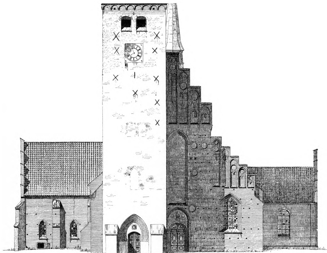
Fig. 21. S. Olai kirke. Vestfacade. 1:300. Tegnet af Christen Larsen 1901 (sml. fig. 15).
