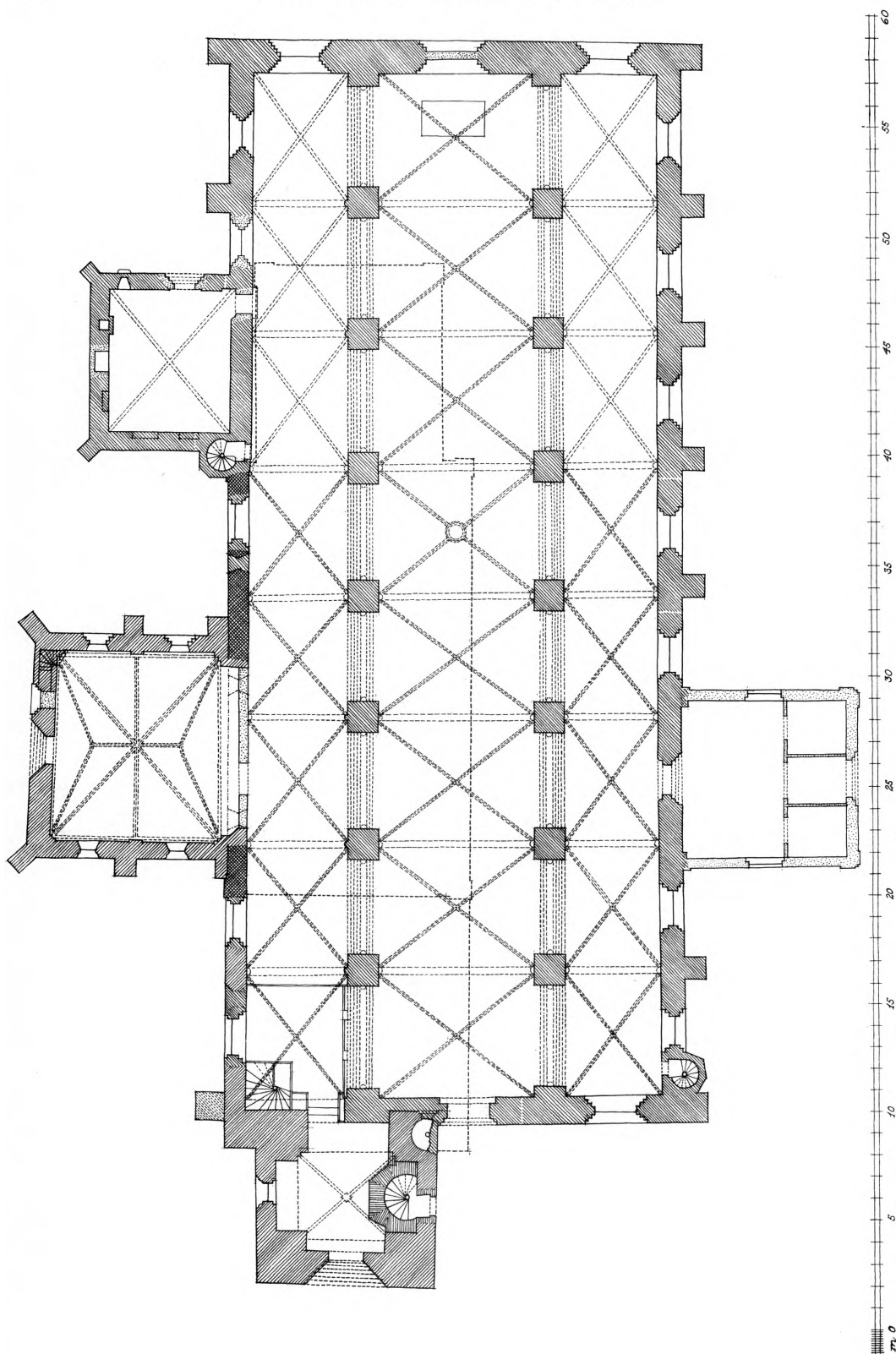
Fig. 16. S. Olai kirke. Plan. 1:300. Øst opad. Tegnet og suppleret af K. de F. L. 1964 på grundlag af opmåling ved Christen Larsen 1901.
