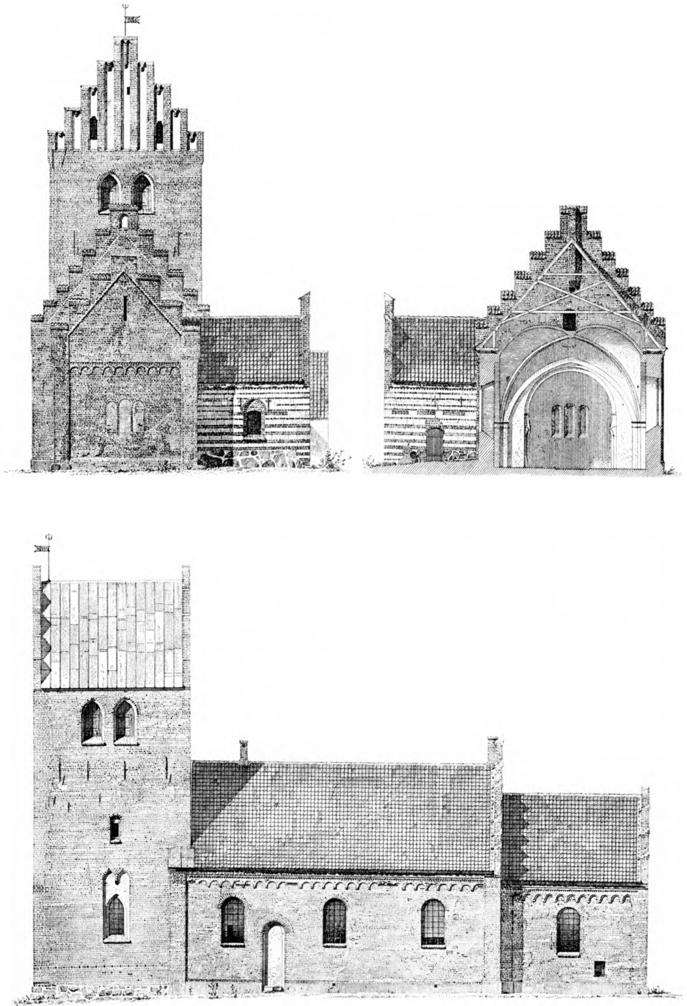
Fig. 3—5. Tikøb. Østfaçade, snit (set mod øst) og sydfaçade. 1:300. Målt af O. V. Koch 1892—93 (jfr. H. Storck og M. Clemmensen: Danske Teglstenskirker).
