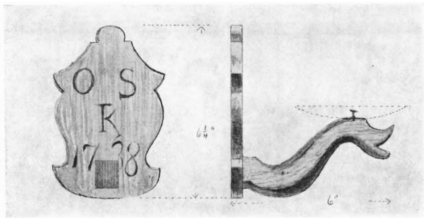
Fig 37. Tikøb. †Lysearm 1738, af træ. Efter tegning af Magnus-Petersen 1884 (p. 712).
