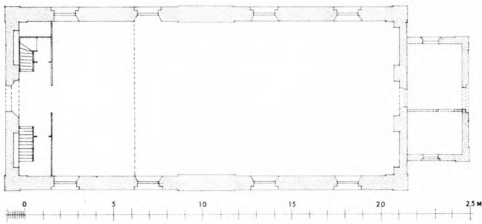
Fig. 2. Hornbæk. Plan. 1:300. Målt af El. M. 1963.
