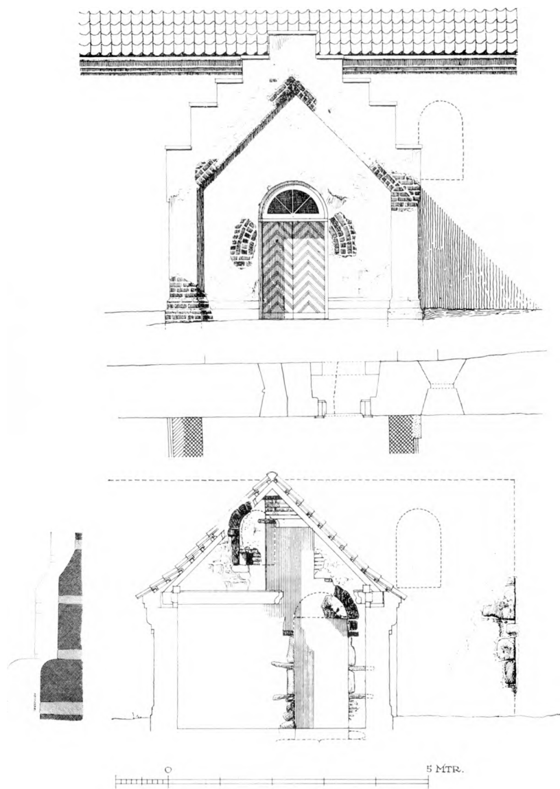
Fig. 6—7. Asminderød. Nordre våbenhus. 1:100. Gavl og snit (set mod skibet) før restaureringen. Forneden til venstre våbenhusets sokkel (skraveret) og sokkelen på Tikøb kor. 1:10. Opmålinger af C. G. Schultz 1930—35.
