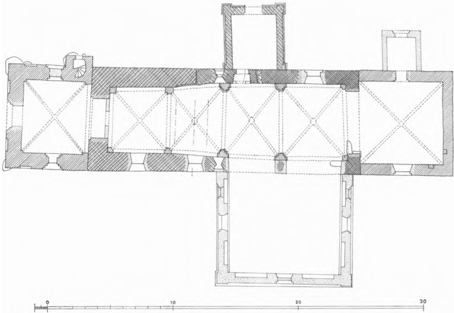
Fig. 2. Asminderød. Plan 1:300. Efter opmåling ved C. G. Schultz 1930 (revideret El.M. 1967).
