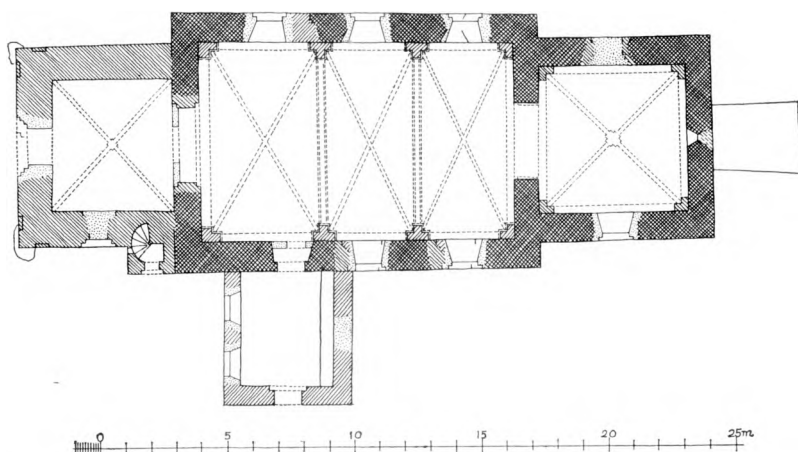
Grønholt. Plan. 1: 300. Målt af C. G. Schultz 1930, suppleret og tegnet af El. M. 1967.
