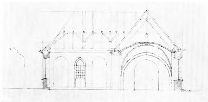
Fig. 6. Esbønderup. Tværsnit i skib og nordre korsarm, set mod øst. 1:300. Målt af elever fra Kunstakademiet o. 1935.
