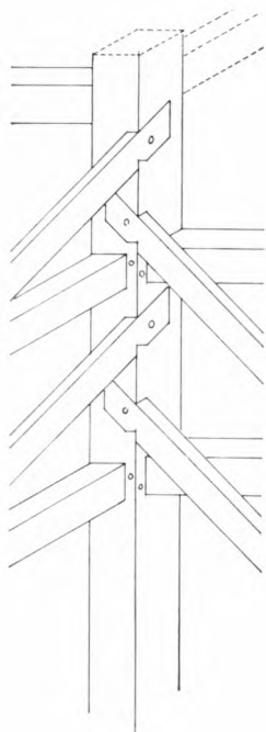
Fig. 3. Esbønderup. Rekonstruktionsskitse af hjørnestolpe i \dagger klok- kehus (p. 1012).
