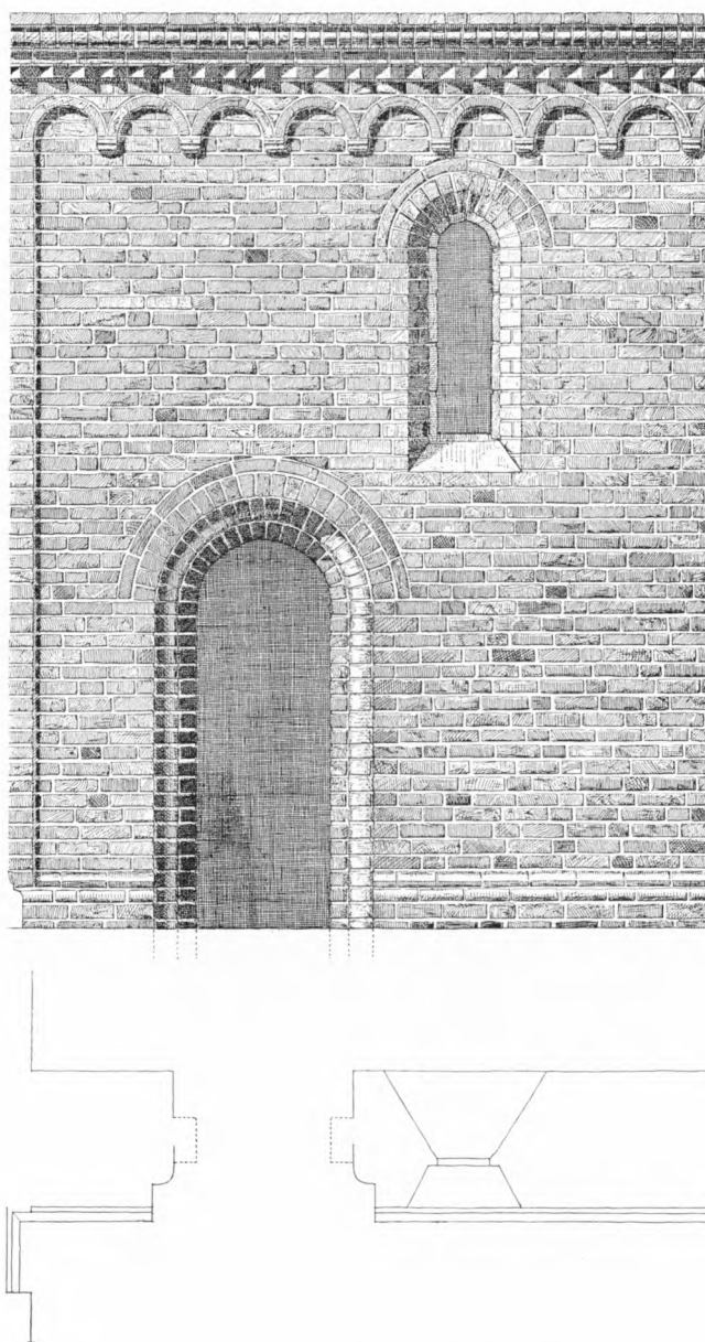
Fig. 5. Soborg. Delvis rekonstrueret udsnit af korets sydmur 1:50. C. G. Schultz 1929 (p. 1104).
