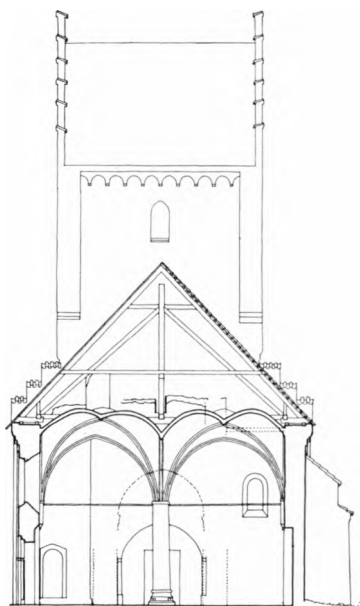
Fig. 7. Søborg. Tværnsnit i skibet set mod vest 1:300; orgeltrappen udeladt.
