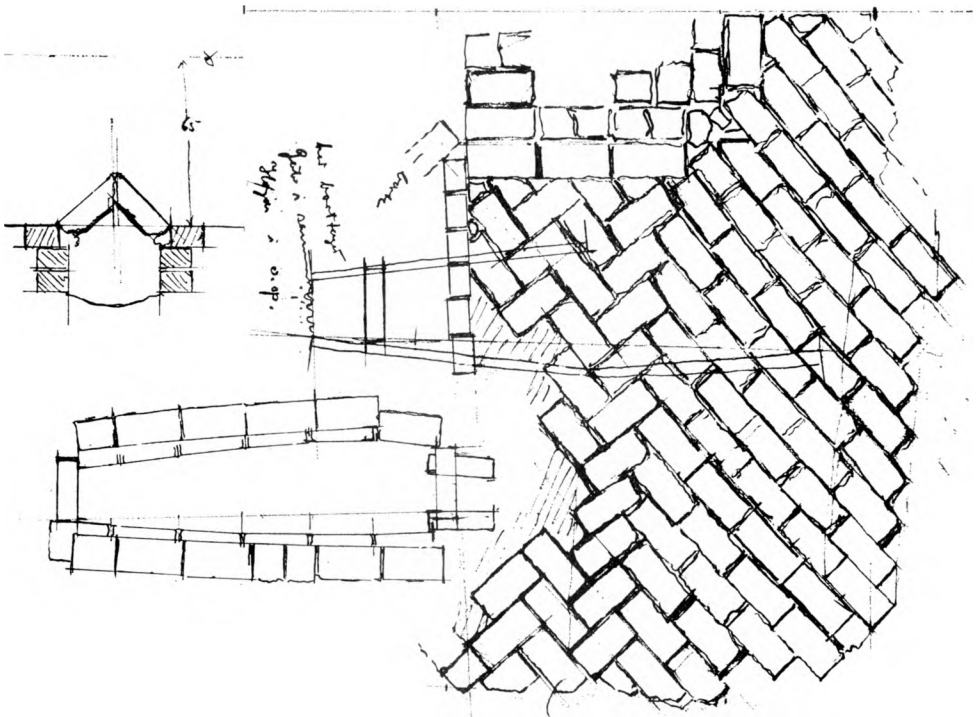
Fig. 18. Soborg. Skitseopmåling 1:30 af middelalderligt teglstengulv og grave i skibets syd-østre hjørne. C. G. Schultz 1939 (p. 1118, 1142).
