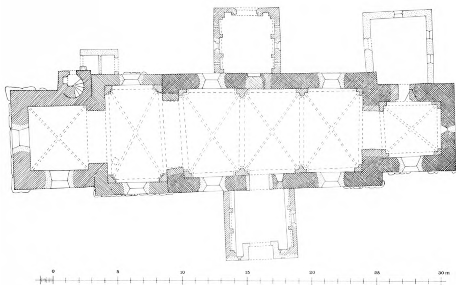
Fig. 2. Græsted. Plan. 1:300. Målt af M. Brahde 1957. Tegnet af H. Reitzel Jensen 1969.
