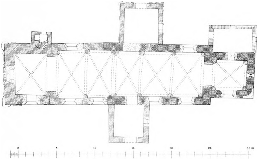
Fig. 2. Helsing. Plan. 1:300. Målt af M. Brahe 1957. Tegnet af Lars Klint 1969.
