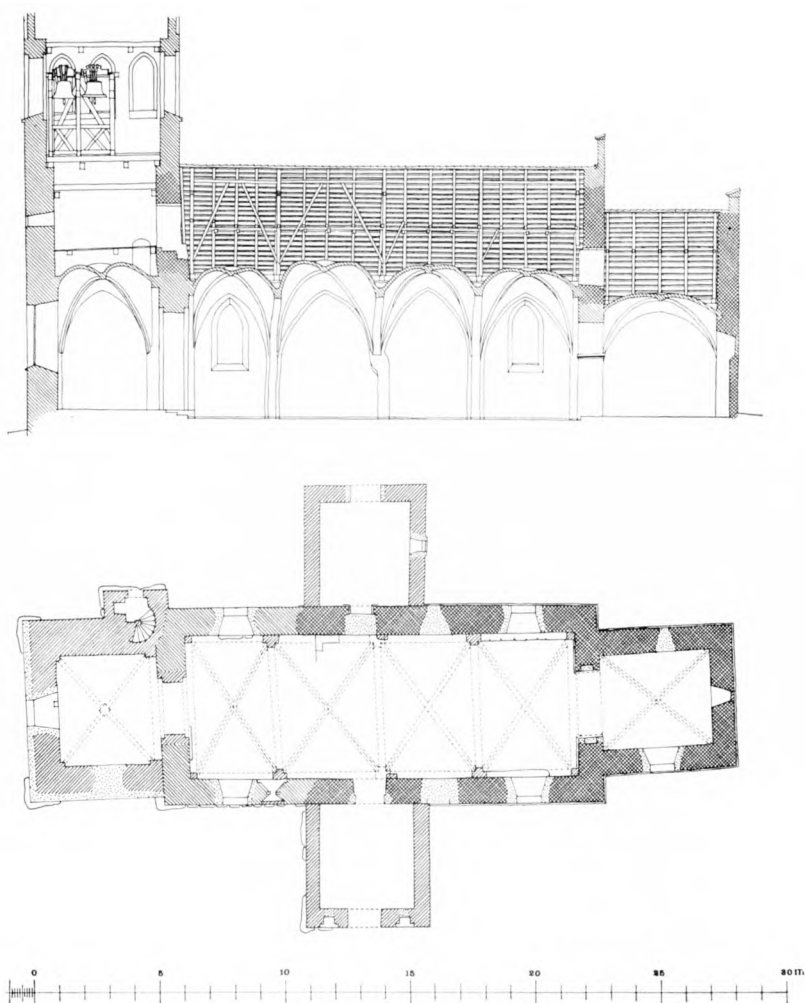
Fig. 2—3. Valby. 2. Langsnit, set mod nord. 1:300. Målt af H. Hoppe, H. Nannestad og H. Ibbo 1942.
