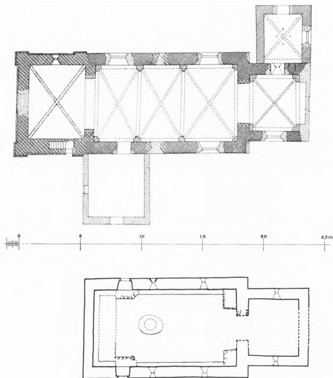
Fig. 2—3. Blistrup. 2. Plan. 1:300. Målt af C. G. Schultz 1930. Suppleret 1969. Tegnet af Lars Klint. 3. Rekonstruktionsplan. 1:300. Tegnet af EL. M. 1969 (p. 1260).
