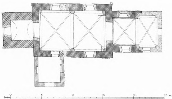
Fig. 2. Annisse. Plan. 1:300. Målt af C. G. Schultz 1935. Suppleret af El. M. 1969.
