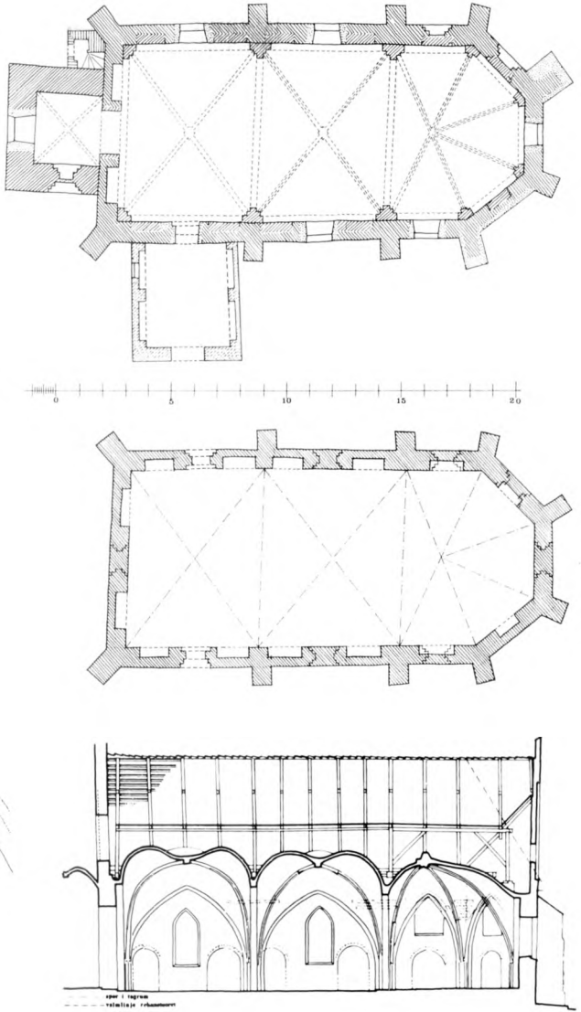
Fig. 2 -5. Alsønderup. 2. Den nuværende plan, målt af H. Brahde 1957. 3. Rekonstruktion af den oprindelige plan (p. 1439). 4. Langsnit set mod nord; prikkede linjer angiver fortændinger og buer til den ældste overhvelvning (p. 1440); målt af Lars Klint og H. Reitzel-Jensen 1969. 1:300. 5. Til venstre. Vindue i korpolygonens nordøstside (p. 1442). 1:100. Målt af H. Hansen 1922. Alt tegnet af El. M. 1970.
