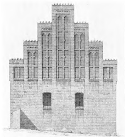
Fig. 5. Melby. Kirkeladens nordgavl. 1:150. Målt af J. B. Løffler 1891 (p. 1611).
