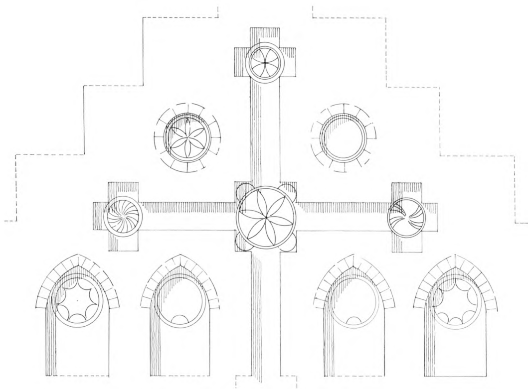
Fig. 7. Melby. Anden vestforlængelse (sml. fig. 8). Blændingsgavl med spor af indridsede dekorationer i blændingernes pudsede bund. 1:50. Tegnet af El. M. 1971 (p. 1614).
