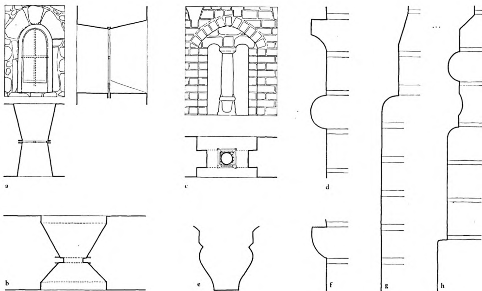
Fig. 2 a—h. Nørre Herlev. Detaljer, a. Vindue i det oprindelige skib (p. 1938). b. Vindue i vestforlængelsen (p. 1938). c. Glamhul i tårnets østmur (p. 1939). d. Kragbånd på skibets hvælpiller (p. 1940). e—f. Ribbeprofil og kragbånd fra østforlængelsens hvælv 1616 (p. 1941). g. Vestforlængelsens sokkel (p. 1938). h. Tårnpillens sokkel (p. 1939). a—c, 1:50. d—h, 1:5. Tegnet af ELM. 1973.
