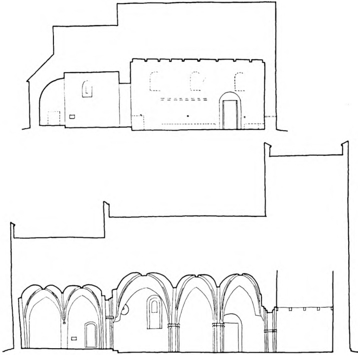
Fig. 5—6. Langsnit (set mod syd). 1:300. 5. Rekonstruktion af kirkens oprindelige udseende (p. 2004.) De stiplede linjer under vinduerne angiver hulrummet efter det formodede hammerbånd (p. 2004.) 6. Kirken efter hvælvenes indbygning og tårnets ombygning (p. 2008).
