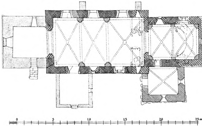
Fig. 2. Uggeløse. Plan. 1:300. Målt af C. G. Schultz 1936, suppleret af El. M. 1972.
