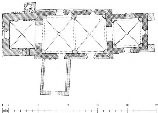
Fig. 2. Gørlose. Plan. 1:300. Målt af C. G. Schultz 1936. Suppleret af El. M. 1972. Tegnet af Jens Hald Jensen 1974.
