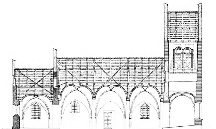
Fig. 3. Græse. Langsnit, set mod syd. 1:300. Tegnet af Einar Jensen 1931 med korrektioner ved Jens Hald Jensen 1974.
