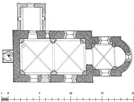
Fig. 2. Sigerslevvester. Plan. 1:300. Målt af G. G. Schultz 1936. Suppleret af El. M. 1973. Tegnet af Jens Hald Jensen 1974.
