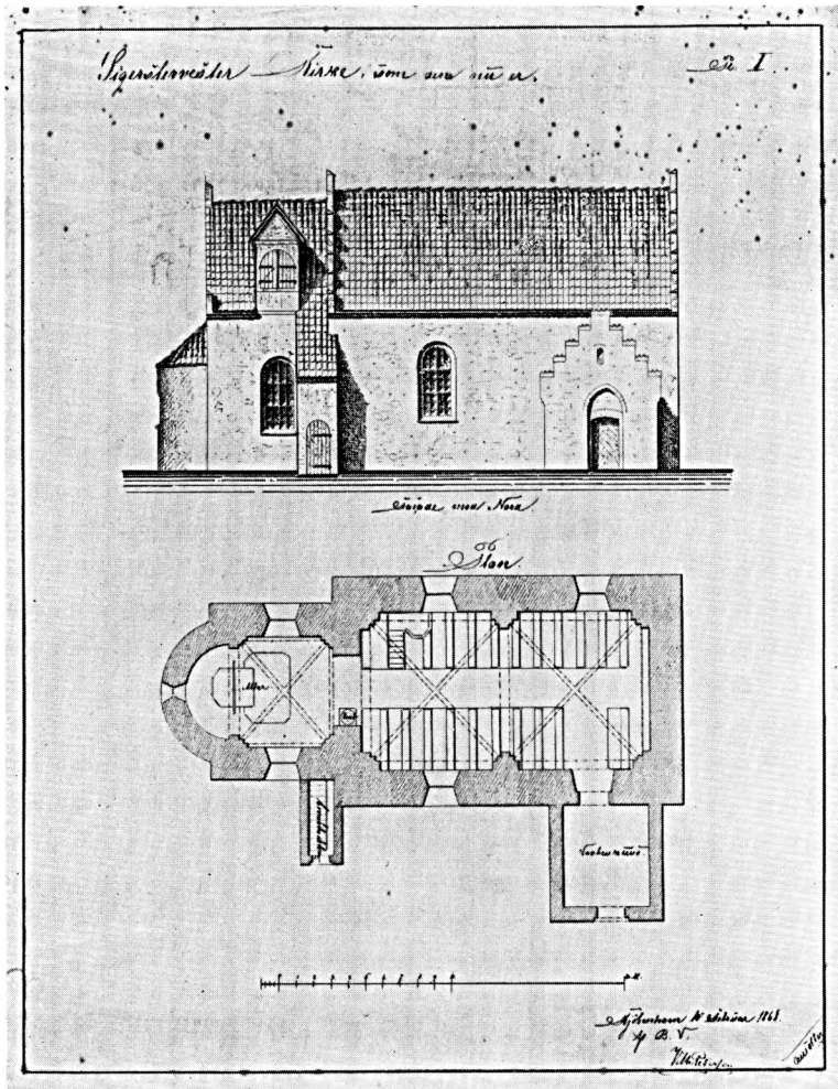
Fig. 4. Sigerslevvester. Plan og opstalt af nordfacade med klokkekviste over koret. 1:300. Opmåling 1868 ved Vilh. Petersen, i Rigsarkivet (p. 2220).
