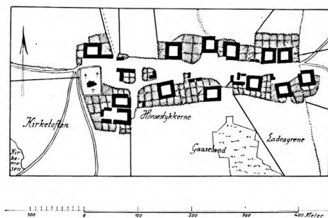
Fig. 10. Sigerslevvester. Landsbyplan 1789.
