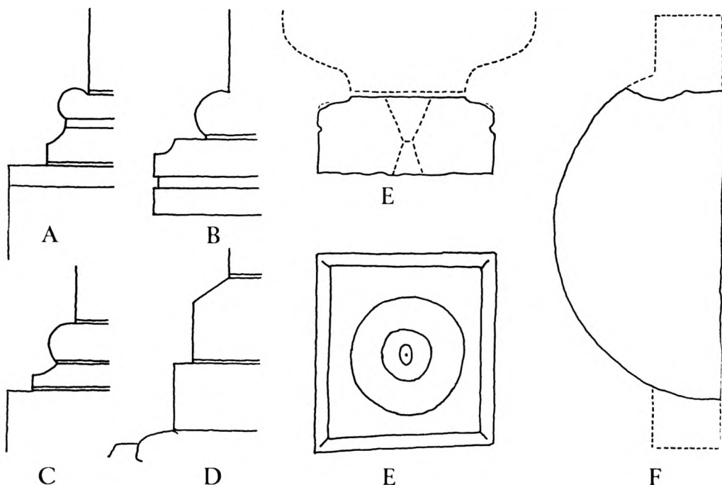
Fig. 10. Jorlunde. Detaljer. 1:20. A sokkel på skib og kor, B sokkel ved skibets sydportal, C sokkel på skibets sydøsthjørne, D sokkel på tårnet ved vestportalen (p. 2238), E fontefod, snit og plan (p. 2268), F tærskelsten ved sakristidøren, genanvendt tympanon (p. 2236). Målt af Hans Stiesdal 1964, tegnet af J. Hald Jensen 1975.
