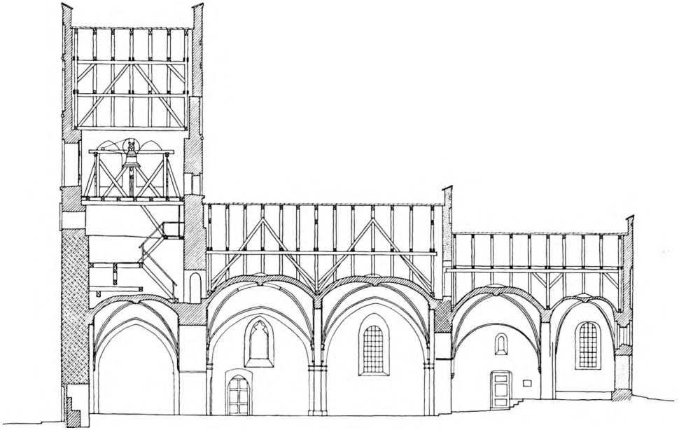
Fig. 2. Jorlunde. Langsnit set mod nord. 1:300. Målt af A. Olsen 1926, suppleret af H. Stiesdal 1964 og J. Hald Jensen 1975. Tegnet af J. Hald Jensen 1975.
