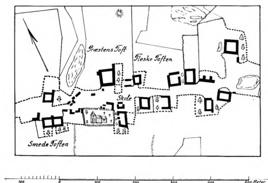
Fig. 30. Jorlunde. Landsbyplan 1807.
