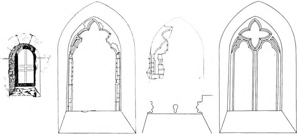
Fig. 4. Jorlunde. Korets nordvindue med oprindelig vinduesramme (p. 2236), målt og tegnet af C. G. Schultz 1938. Nordvindue i skibets vestfag (p. 2244), målt af H. Stiesdal 1964 (indvendig) og H. Schmidt 1963 (udvendig og plan). Rekonstruktion tegnet af J. Hald Jensen 1975. 1:50.
