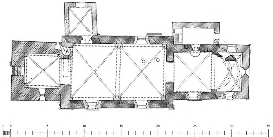
Fig. 3. Jorlunde. Plan. 1:300. Målt af C. G. Schultz 1938 og suppleret af H. Stiesdal 1964. Tegnet af J. Hald Jensen 1975.
