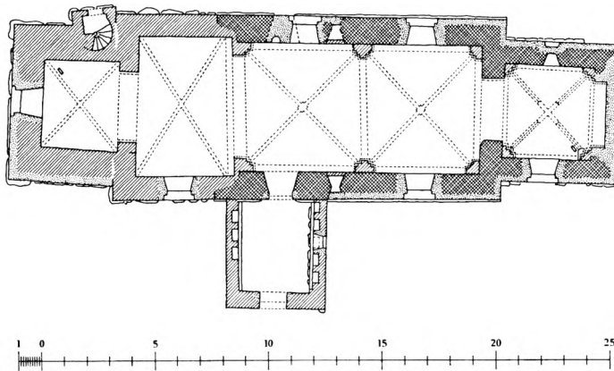
Fig. 3. Snostrup. Plan. 1:300. Målt af C. G. Schultz 1936. Tegnet af Jens Hald Jensen 1975.
