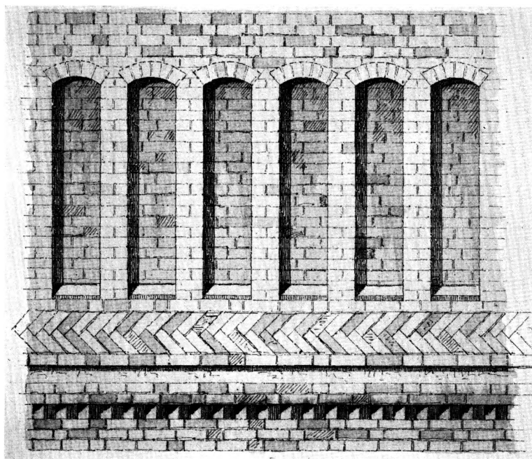
Fig. 6. Krogstrup. Udsnit af vestforlængelsens gavl med blændingsdekoration. 1:50. Tegning i Nationalmuseet, signeret J. B. Løffler 1873—74 (p. 2730).
