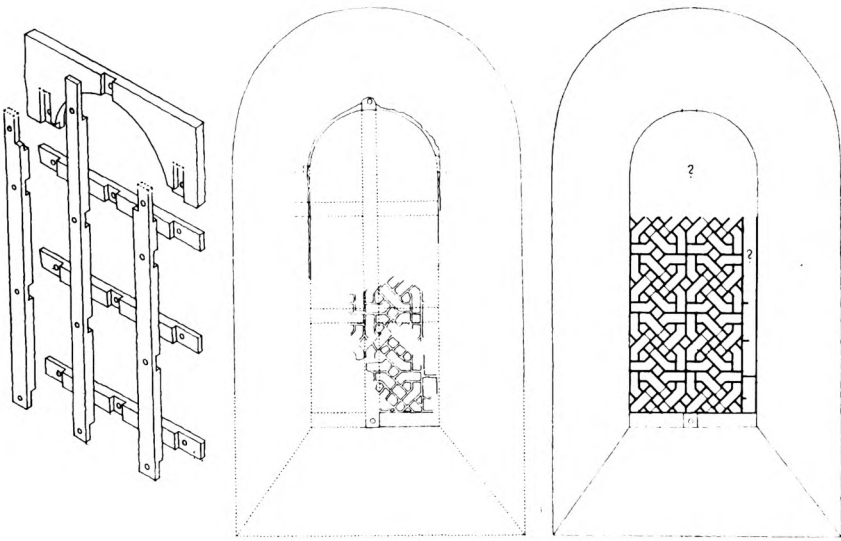
Fig. 3 a—c. Krogstrup. Romansk vindue i skibets nordside. 1:25. Tegnet af Erik Hansen 1962. a. Rekonstruktion af oprindelig træramme (p. 2728). b. Indvendig opstalt med aftryk af glasmosaik, c. Rekonstruktion af glasmosaikken (p. 2735).
