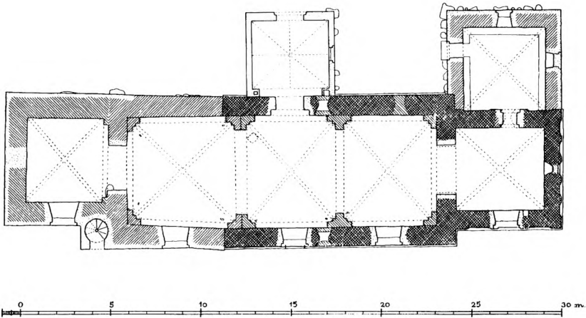
Fig. 2. Krogstrup. Plan. 1:300. Målt af C. G. Schultz 1935, tegnet af Henrik Jacobsen 1977.
