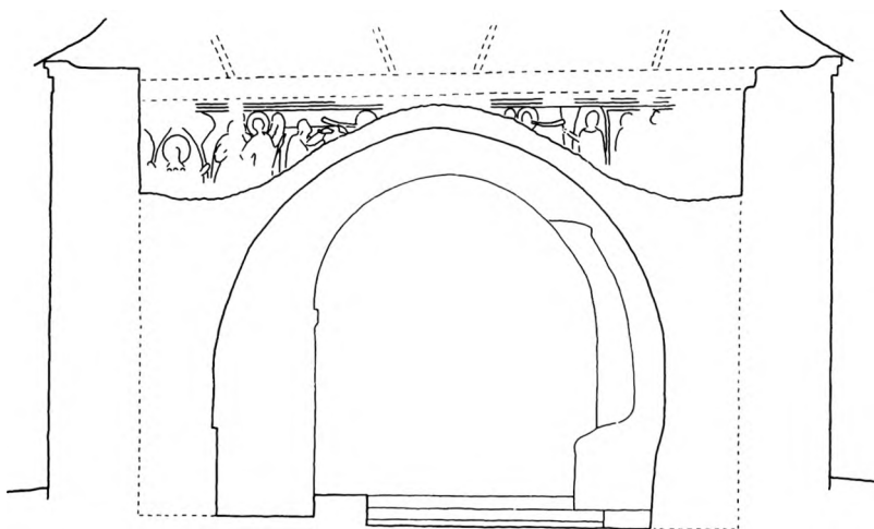
Fig. 9. Ferslev. Tværnsnit ved triumfurens vestside med kalkmaleriudsmykning. 1:100. Målt af Henrik Jacobsen og H. J., tegnet af førstnævnte 1977 (p. 2764).
