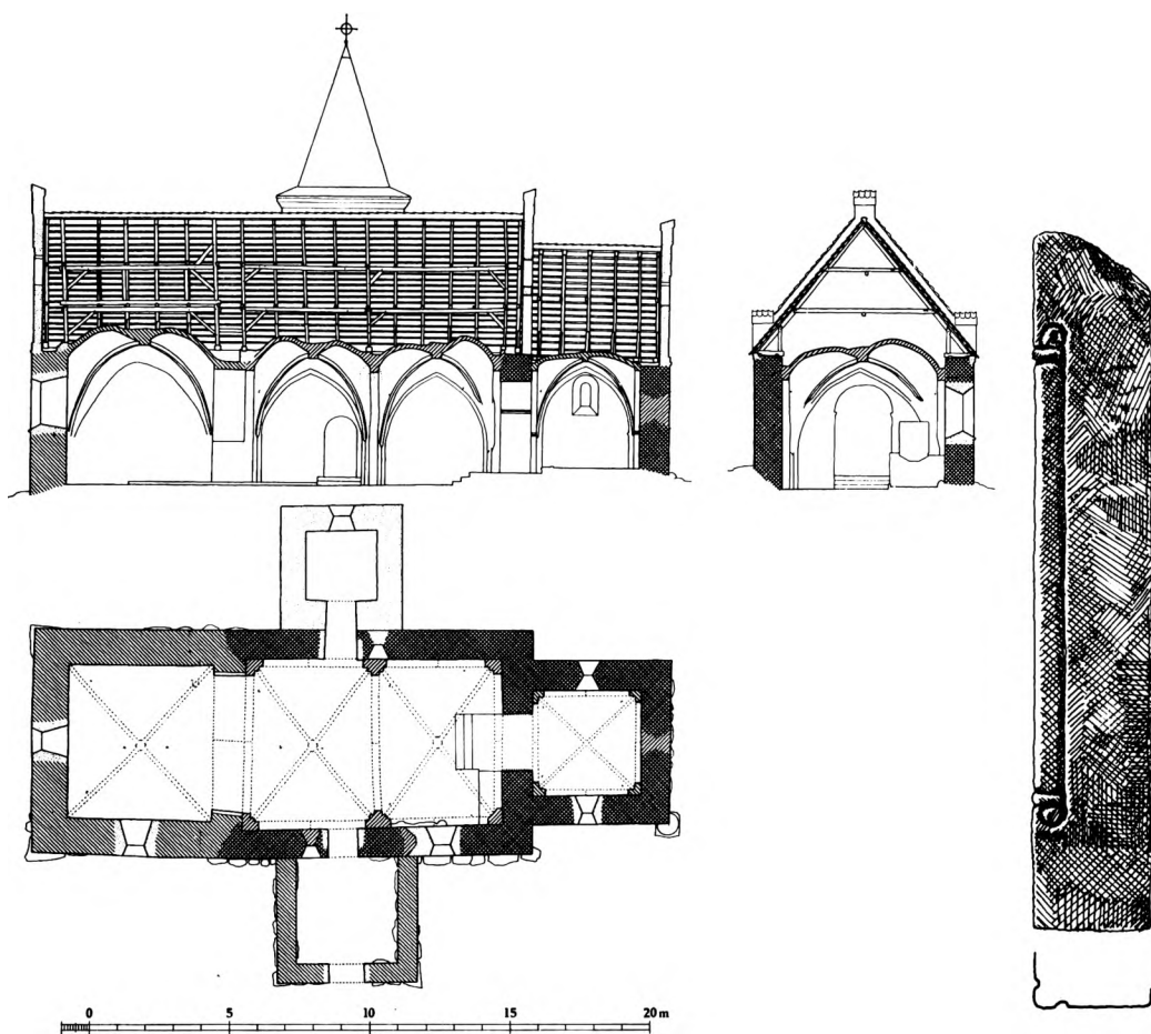
Fig. 4—5. Vellerup. 4. Snit og plan. 1:300. Målt og tegnet af Henrik Jacobsen 1973 med korrektioner 1976. 5. Karmsten i norddøren. 1:20 (p. 2781). Henrik Jacobsen og K. de F. L. 1976.
