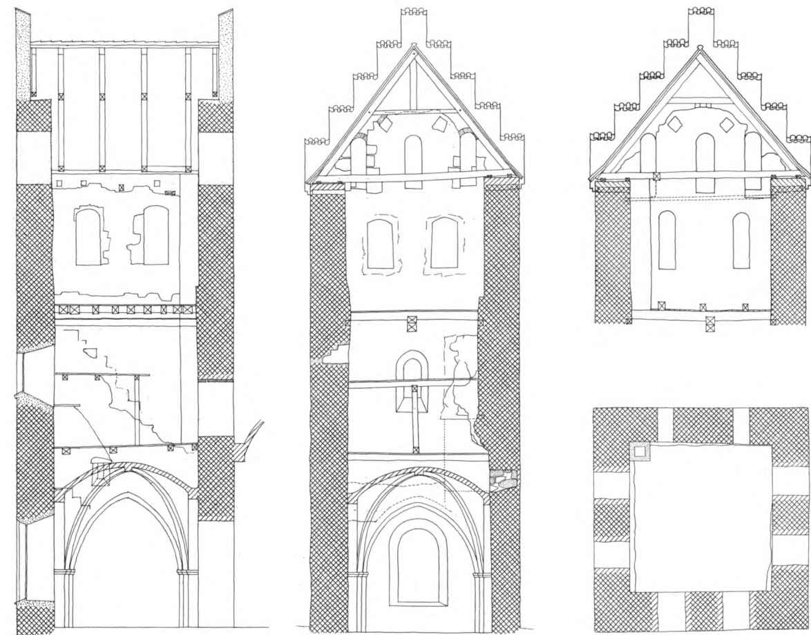
Fig. 5 a-d. Plan og tværnsnit af tårn. a-c. Tværnsnit set mod nord, vest og øst. d. Plan af klokkestokværk. 1:150. a, b og d er målt og tegnet af E. Hansen m.fl. 1963, c af S. Rassov og M. Thon 1978. — Plan and cross-sections of the tower. a-c. Cross-sections to the north, west and east. d. Plan of belfry.
