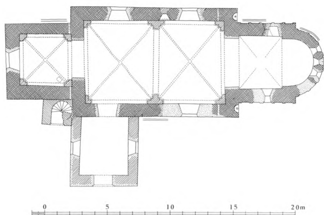
Fig. 2. Plan. 1:300. Målt af MB 1959, tegnet af HJ 1979. Signaturforklaring s.9. — Ground-plan. Key on p. 9.
