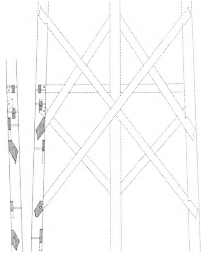
Fig. 23. Forslag til anbringelse af egebjælke fra klokkestokværkets gulv i fritstående klokkehus (s.86). 1:75. Opmåling og rekonstruktionstegning ved E. Hansen m.fl. 1963. — Proposed location of oak beam in a free-standing bell-tower, now re-used among the floor beams of the tower.
