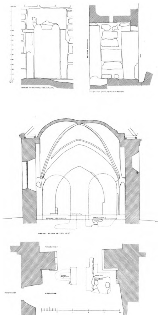
Fig. 2-4. 2. Plan. 1:300. Målt af I. Arthur-Nielsen 1958, tegnet af HJ 1979. Signaturforklaring s. 9. — Ground-plan. Key on p.93. Opstalt og snit af oprindelig åbning i korets vestgavl. 1:50 (s. 180). Målt 1958 og tegnet 1963 af I. Arthur-Nielsen. — Elevation and cross-section of original opening in the west gable of the chancel. 4. Plan og snit i skibets vestende med levn af oprindelig tårnarkade. 1:150 (s. 182). Målt 1950 og tegnet 1963 af I. Arthur-Nielsen. — Cross-section of the western part of the nave showing remains of original arcade between nave and tower.
