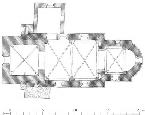
Fig. 2. Plan. 1:300. Målt af MB 1959, tegnet af HJ 1979. Signaturforklaring s.9. — Ground-plan. Key on p. 9.
