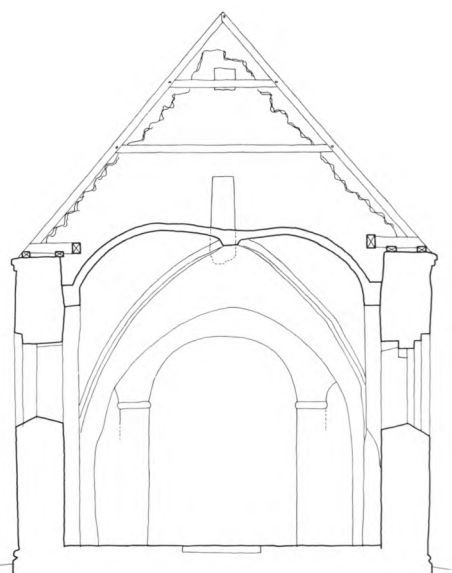
Fig. 3. Tværnsnit i skibet, set mod triumfmuren. 1:150. Målt af Kirsten Kildegaard Petersen, Thomas A. Sørensen og HeJ 1978, tegnet af HJ 1979. — Cross-section of the nave seen towards the east wall of the nave.
