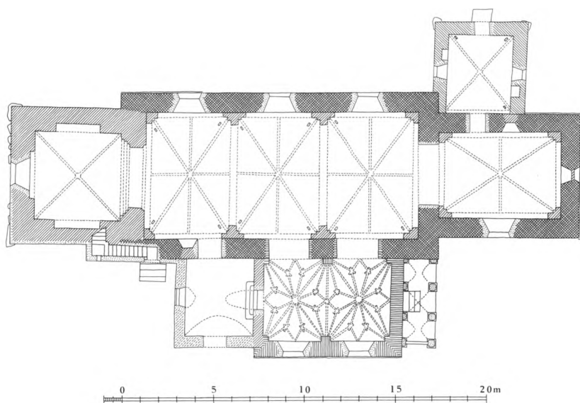
Fig. 2. Plan. 1:300. Målt af MB 1959, tegnet af HJ 1979. Signaturforklaring s. 9. — Ground-plan. Key on p.9.
