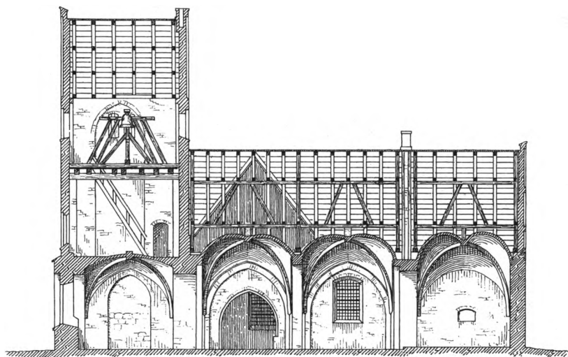
Fig. 4. Længdesnit. 1:300. Målt og tegnet af F. C. C. Hansen 1893. Efter Løffler: Sorø Landsbykirker. - Longitudinal section.
