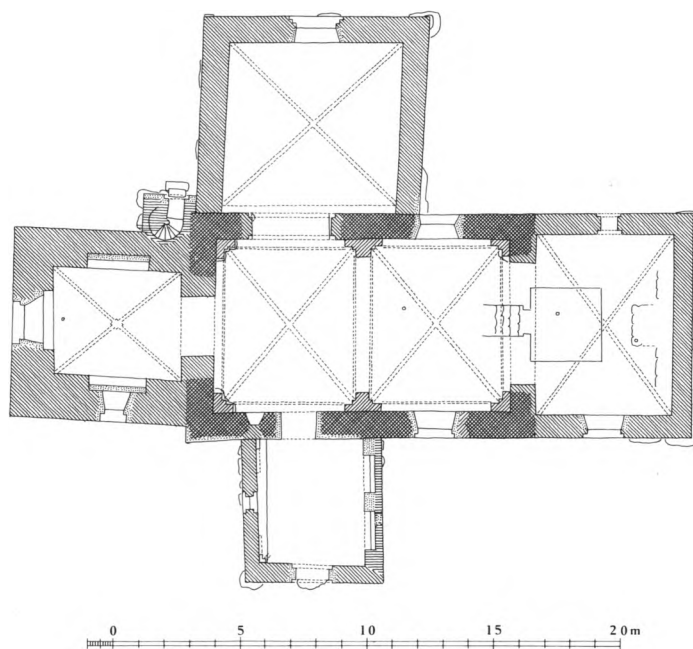
Fig. 2. Plan. 1:300. Målt af MB 1959, suppleret af ELM 1961, revideret og tegnet af HJ 1981. Signaturforklaring s. 9. - Ground-plan. Key on p.9.
