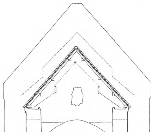
Fig. 3-4. 3. Triumfgavlens, set fra øst med spor efter korets ældste tag (s. 496). Triumfgavlens oprindelige kam er angivet med stiplede linje. 4. Skibets vestgavl, set fra tårnrum (s. 491). 1:150. Målt af Flemming Beyer, Tony B. Munch og Jørgen G. Nielsen 1977, tegnet af Beyer 1981. - 3. West gable of the chancel with traces of the earliest chancel roof. The original roof slope is indicated by dots. 4. West gable of the nave seen from the tower.
