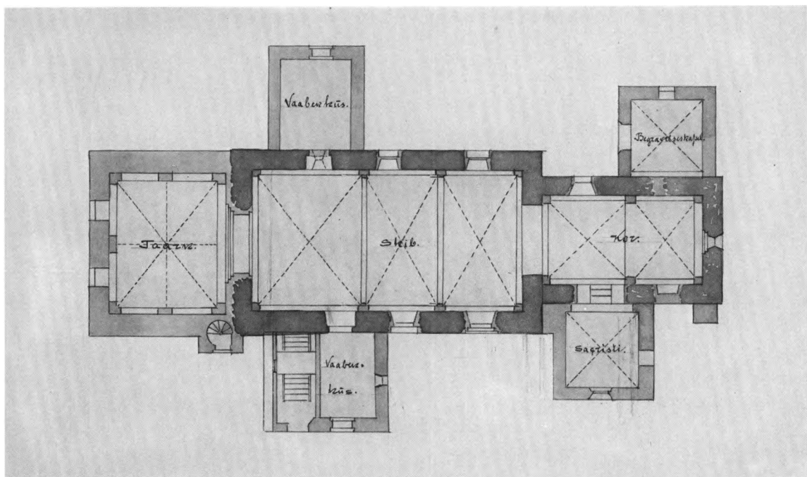
Fig. 7. Plan. 1:300. Tegnet af Aage H. Mathiesen 1894. Bemærk søndre våbenhus med indgang til herskabs-pulpitur, inden ombygningen 1910-11 (s. 492). - Plan. Notice the south porch with entrance to the manorial pew, before rebuilding in 1910-11.
