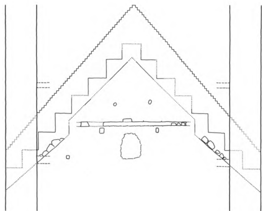
Fig. 3-4. 3. Triumfgavlens, set fra øst med spor efter korets ældste tag (s. 496). Triumfgavlens oprindelige kam er angivet med stiplede linje. 4. Skibets vestgavl, set fra tårnrum (s. 491). 1:150. Målt af Flemming Beyer, Tony B. Munch og Jørgen G. Nielsen 1977, tegnet af Beyer 1981. - 3. West gable of the chancel with traces of the earliest chancel roof. The original roof slope is indicated by dots. 4. West gable of the nave seen from the tower.
