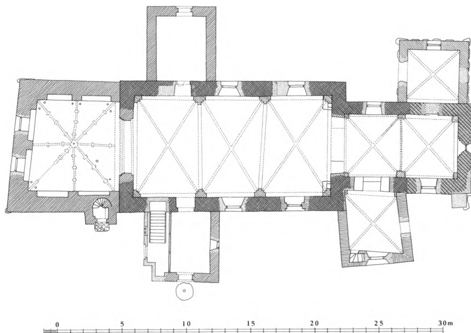
Fig. 2. Plan. 1:300. Målt af MB 1960, suppleret af Flemming Beyer m.fl. og tegnet af HJ 1981. Signaturforklaring s. 9. - Ground-plan. Key on p. 9.
