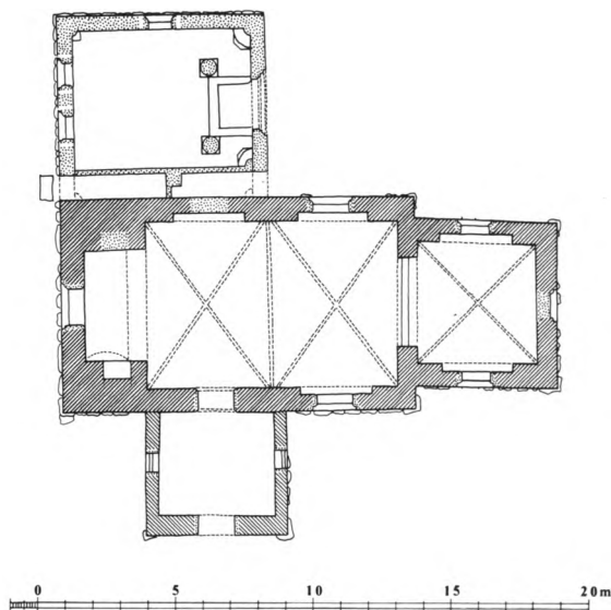
Fig. 2. Plan. 1:300. Målt af MB i 1960, tegnet af Marianne Nielsen 1983. Signaturforklaring s. 9. - Ground-plan. Key on p. 9.
