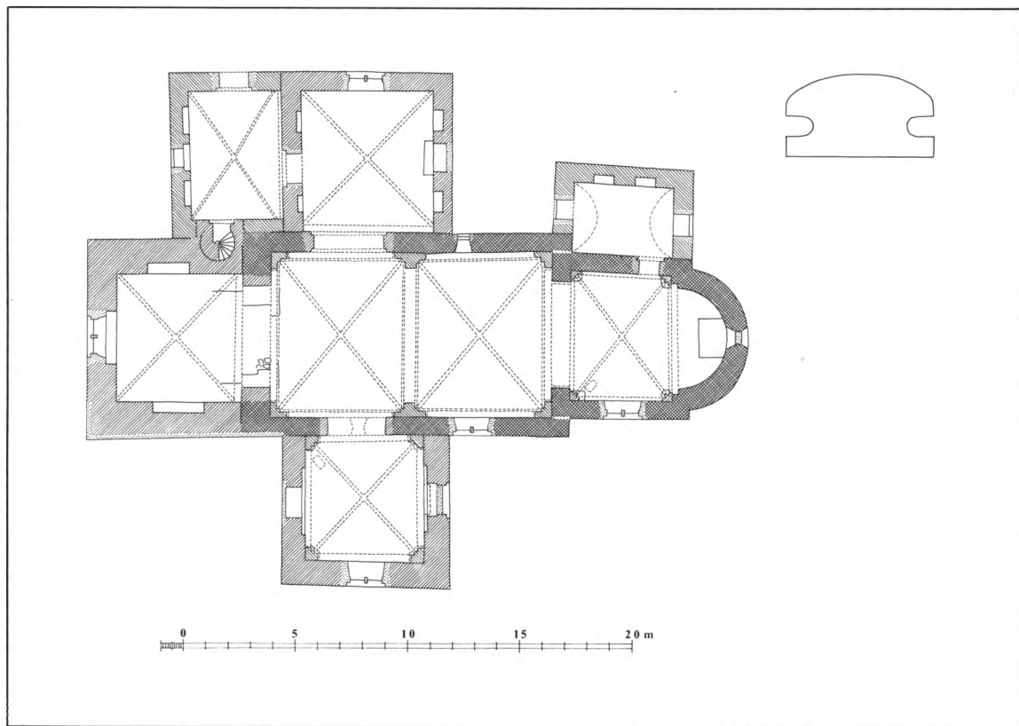
Fig. 3-3a. 3. Plan. 1:300. Målt af Paul Momme 1925, suppleret og korregeret af E1M 1966 og HJ 1978; tegnet af Marianne Nielsen 1983. Signaturforklaring s. 9. 3a. Tværsnit af stavplanke, jfr. fig. 4 (s. 896). 1:10. - 3. Ground-plan. Key on p.9. 3a. Cross-section of stave plank.
