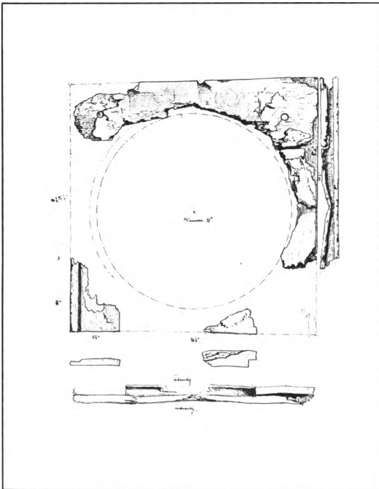
Fig. 5. *Rester af egetræsramme fra apsidens cirkelvindue, jfr. fig. 13 (s. 897). 1:15. Målt og tegnet af Eigil Rothe 1907. - Remains of oak frame from the circular window in the apse.
