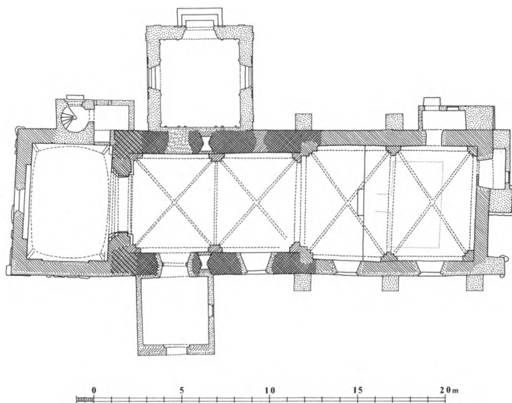
Fig. 2. Plan. 1:300. Målt af MB 1966, suppleret af HJ og tegnet af Marianne Nielsen 1984. Signaturforklaring s. 9. - Ground-plan. Key on p. 9.
